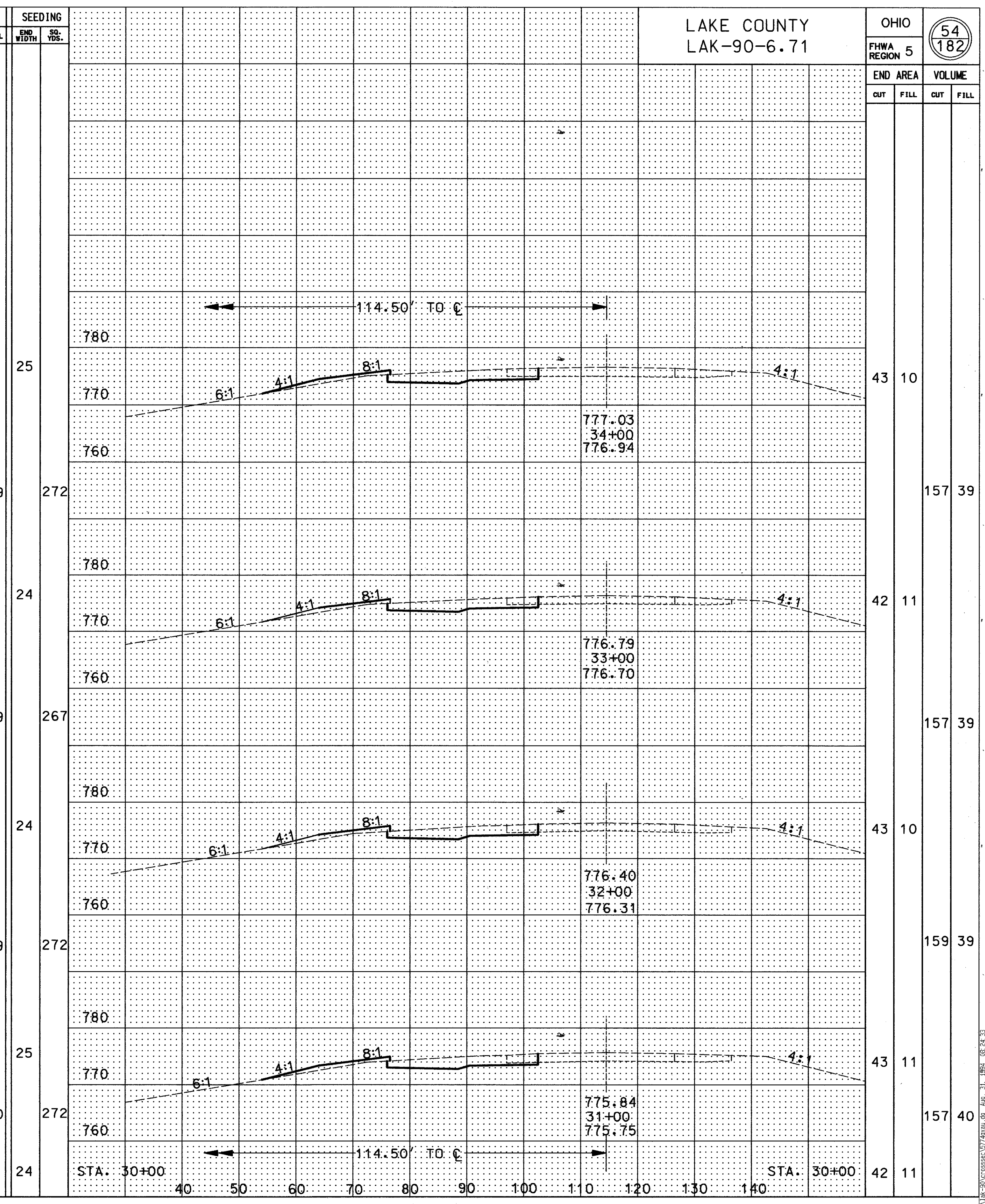
CROSS SECTIONS STA. 31+00 TO STA. 34+00 (WB) & STA. 31+00 TO STA. 34+00 (EB)
