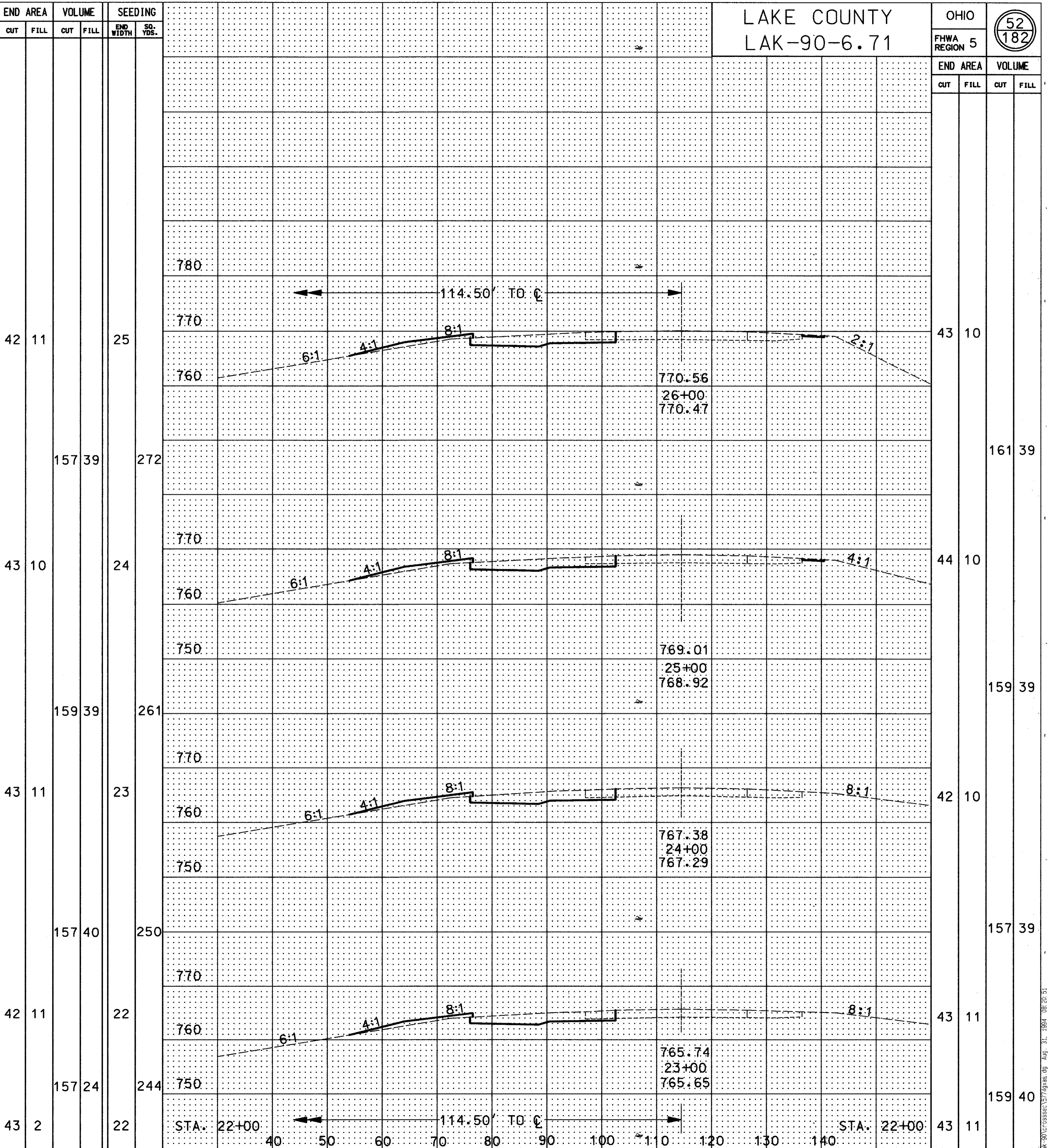
CROSS SECTIONS STA. 23+00 TO STA. 26+00 (WB) & STA. 23+00 TO STA. 26+00 (EB)
