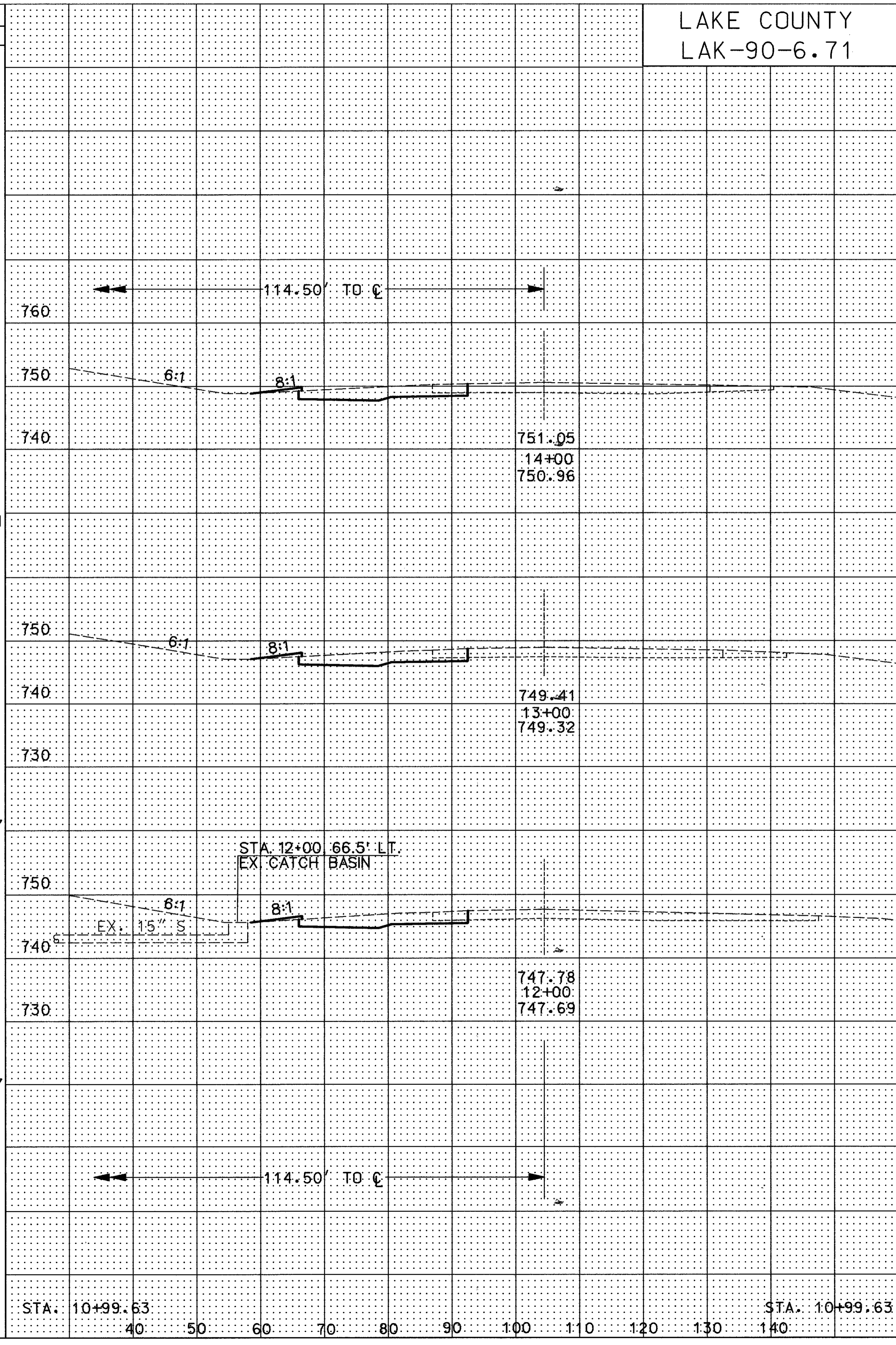
CROSS SECTIONS STA. 12+00 TO STA. 14+00 (WB) & STA. 12+00 TO STA. 14+00 (EB)
