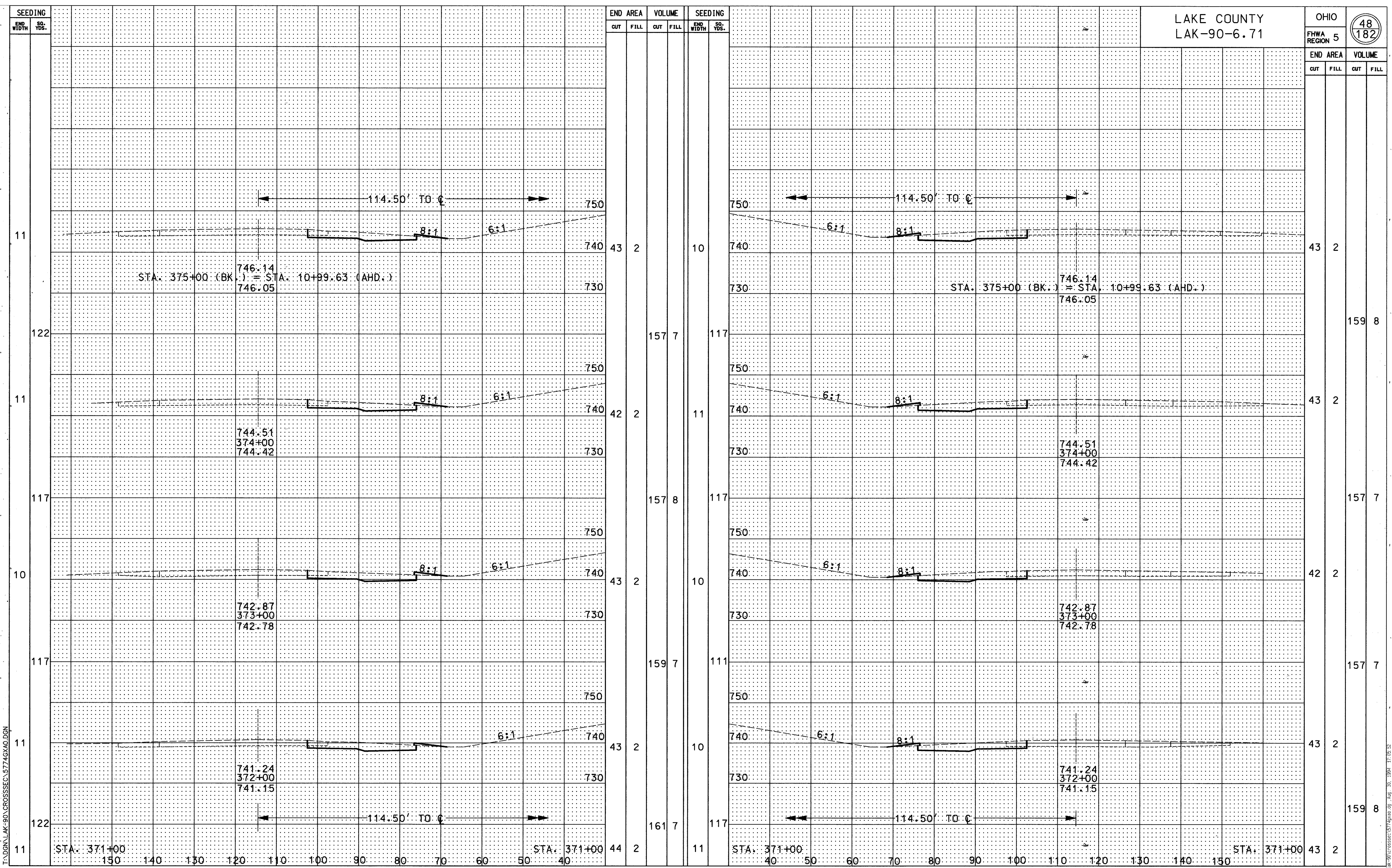
CROSS SECTIONS STA. 372+00 TO STA. 375+00 (WB) & STA. 372+00 TO STA. 375+00 (EB)
