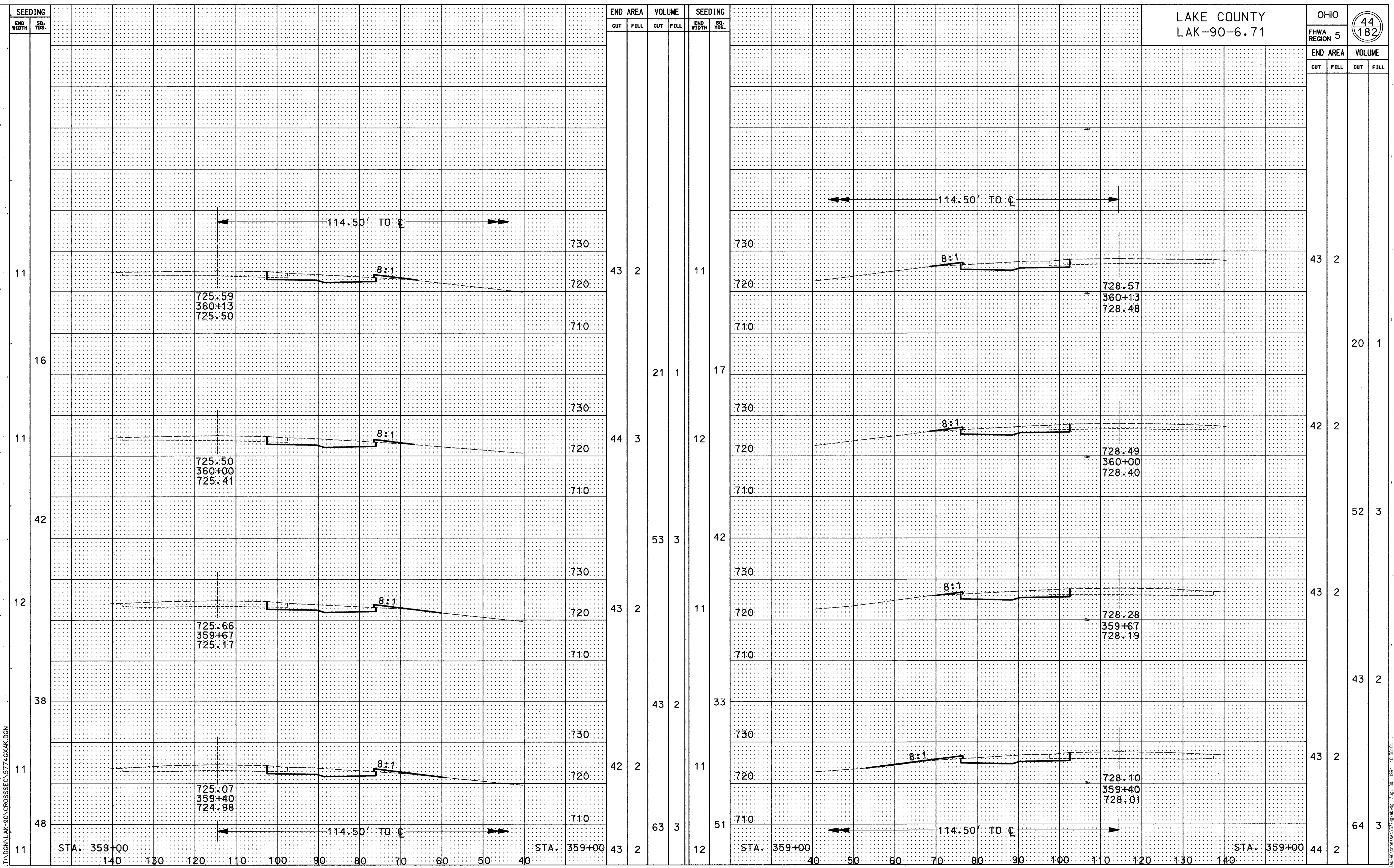
CROSS SECTIONS STA. 359+40 TO STA. 360+13 (WB) & STA. 359+40 TO STA. 360+13 (EB)
