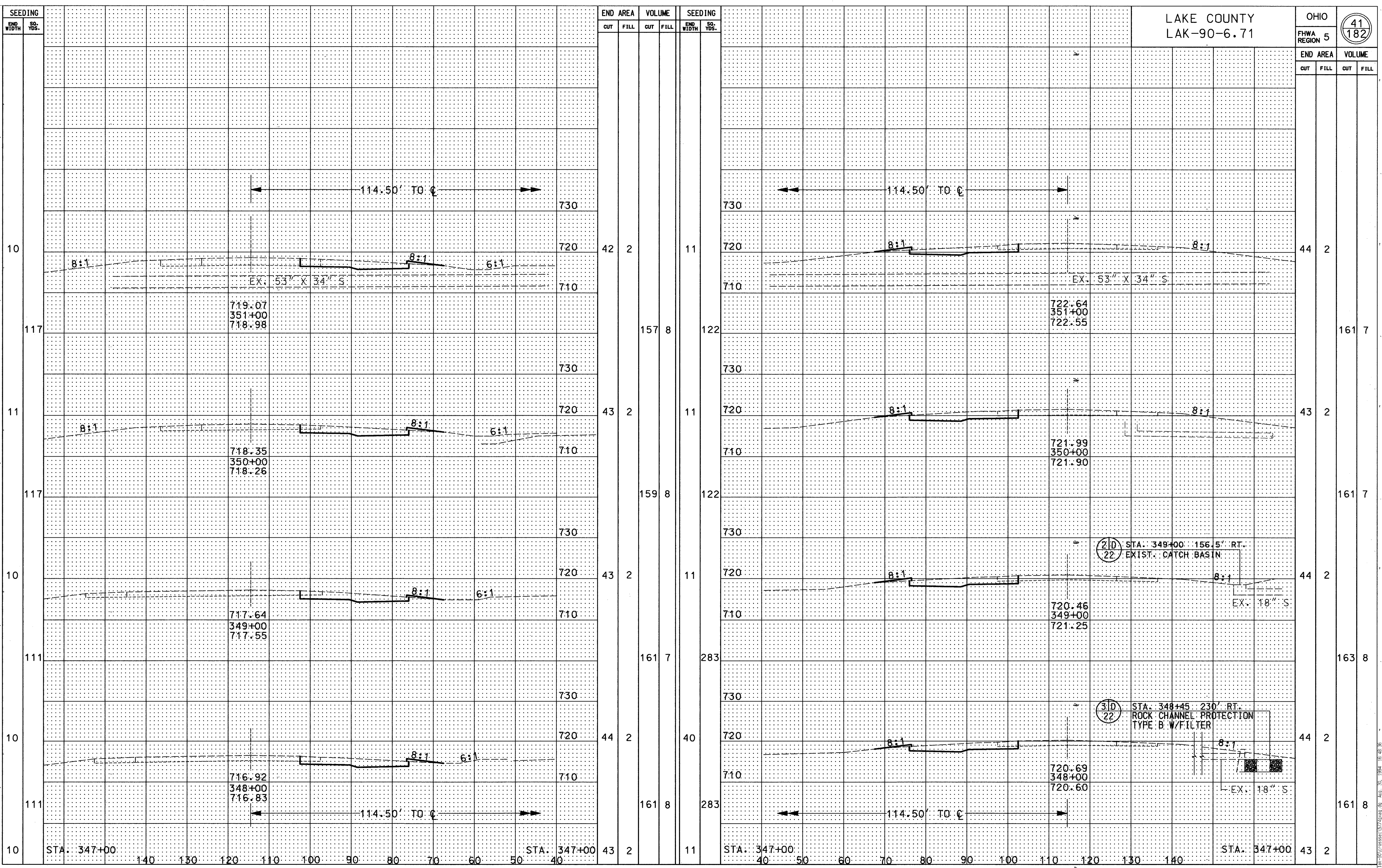
CROSS SECTIONS STA. 348+00 TO STA. 351+00 (WB) & STA. 348+00 TO STA. 351+00 (EB)
