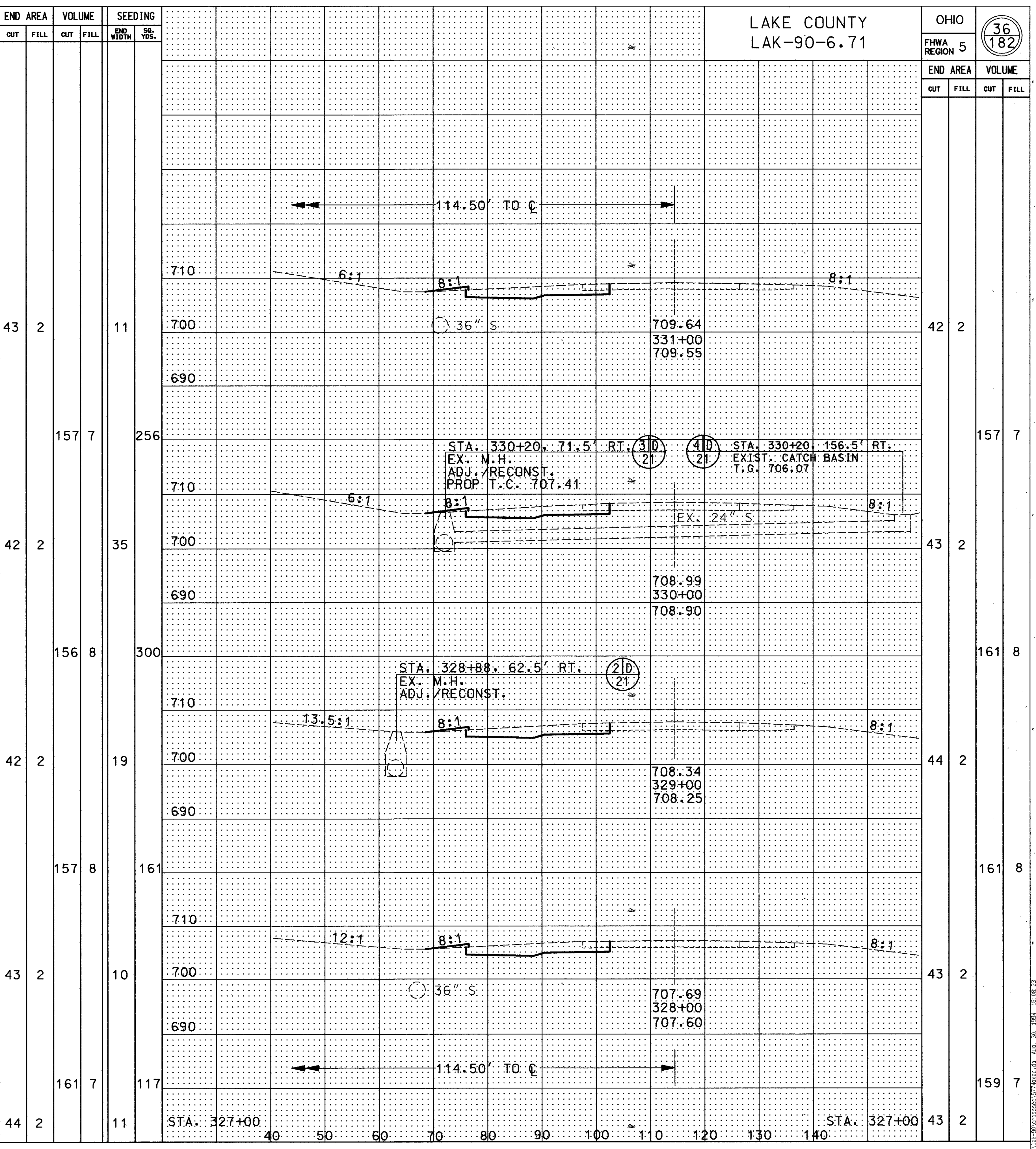
CROSS SECTIONS STA. 328+00 TO STA. 331+00 (WB) & STA. 328+00 TO STA. 331+00 (EB)
