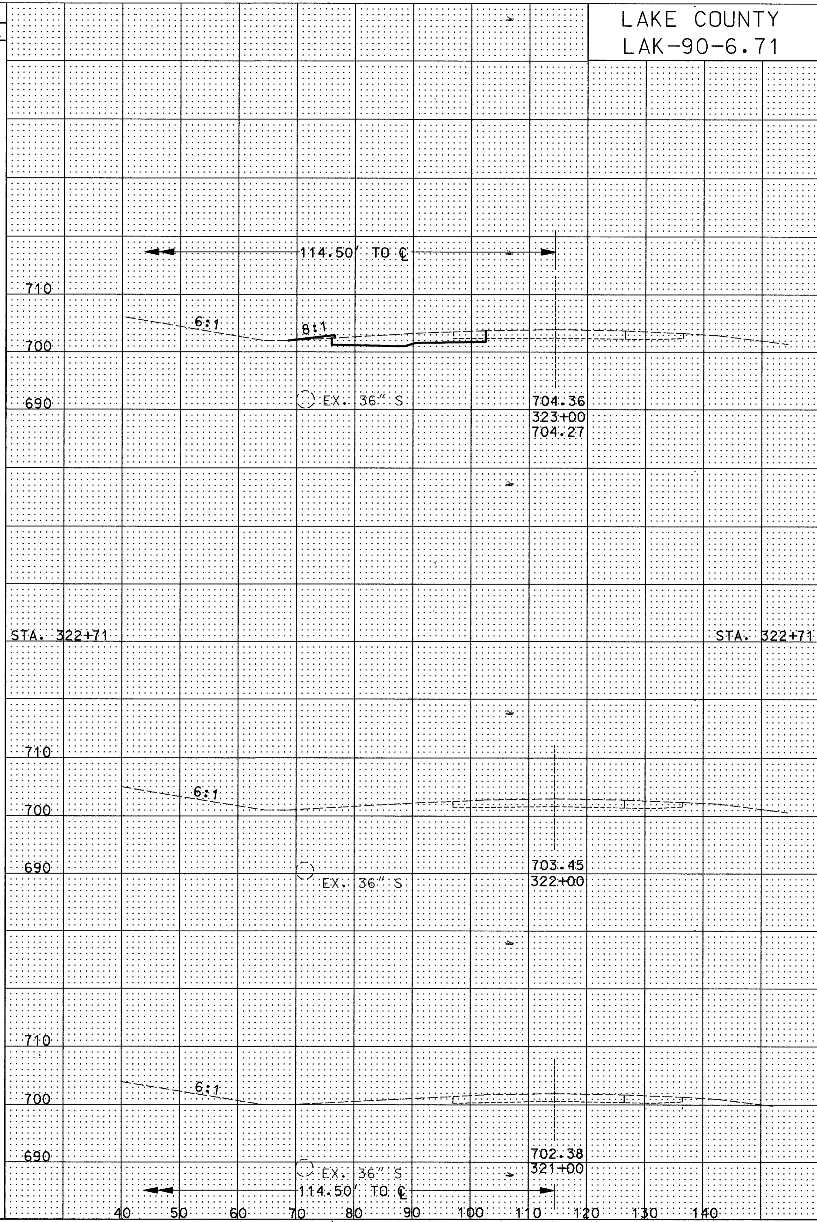
CROSS SECTIONS STA. 321+00 TO STA. 323+00 (WB) & STA. 321+00 TO STA. 323+00 (EB)
