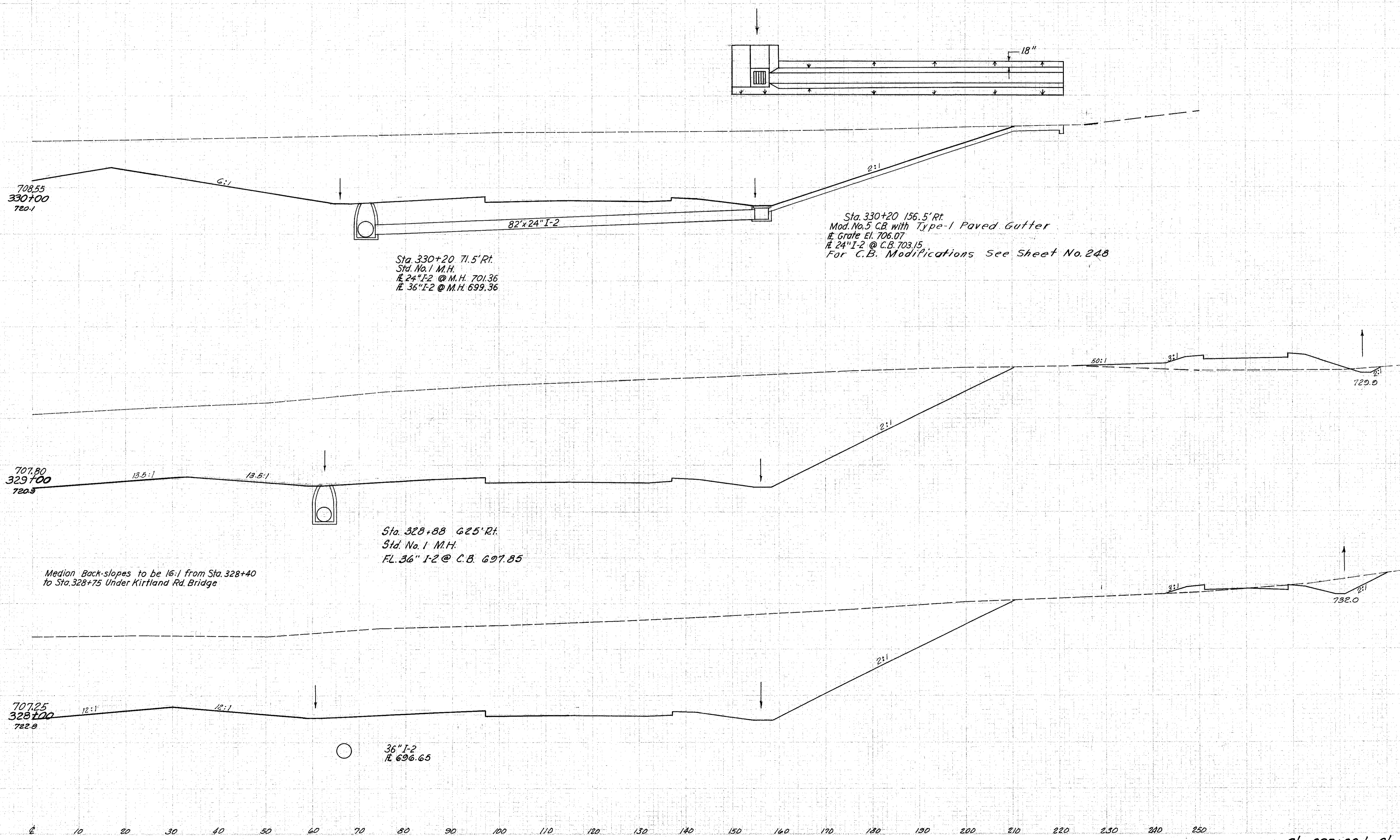
Sta. 328+00 to Sta. 330+00 Rt. 2
