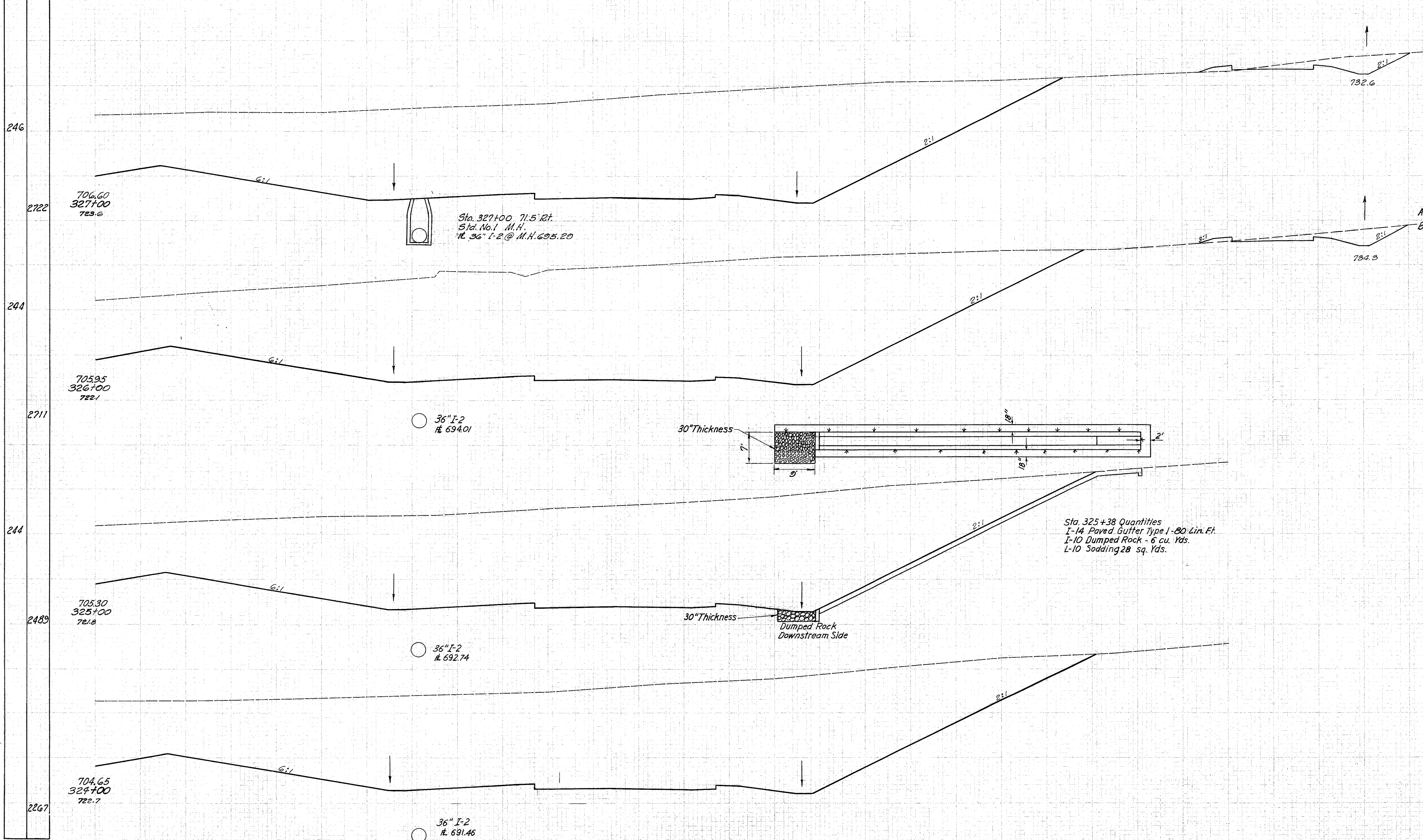
Sta. 324+00 to Sta. 327+00 Rt. 4
