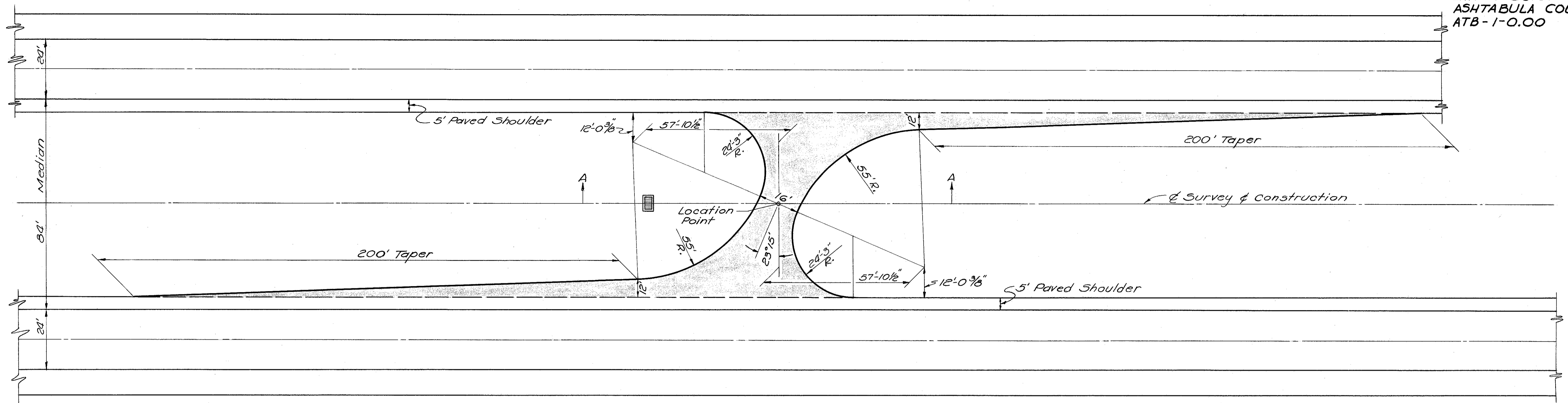
PLAN Scale: 1" = 20'
