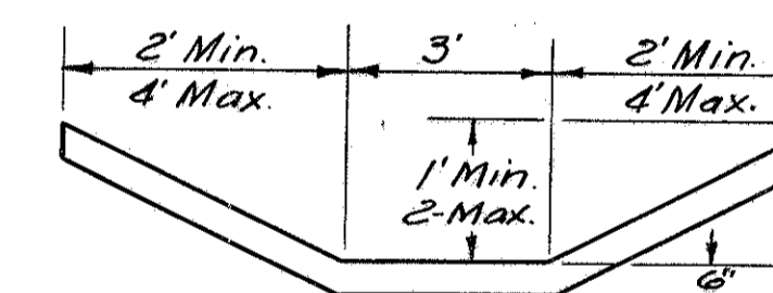
SECTION B-B TYPE "A" RIPRAP
