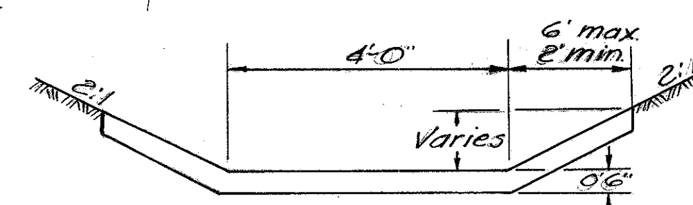
SECTION B-B TYPE "A" RIPRAP
