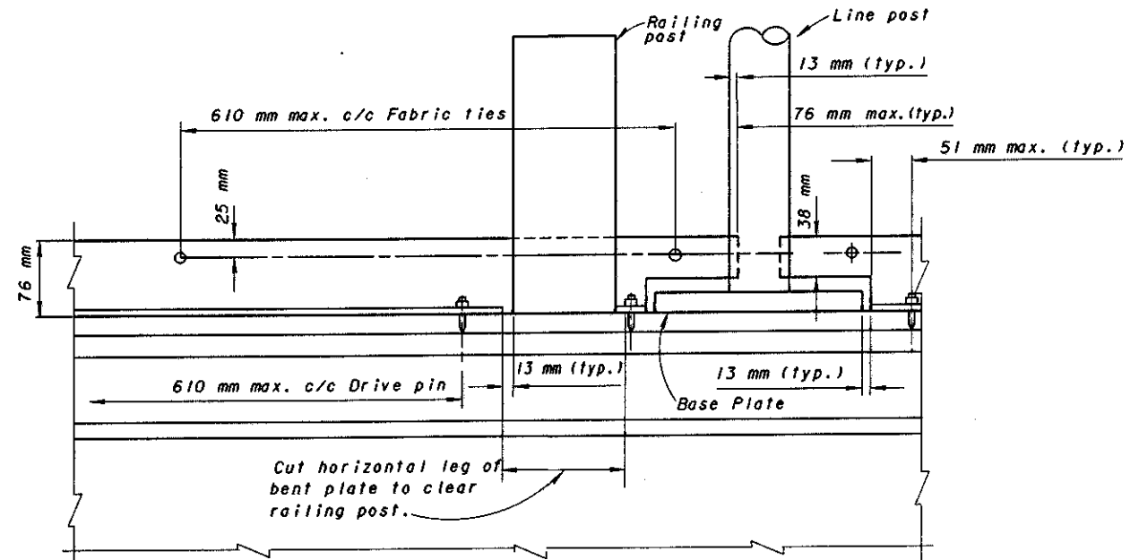
VIEW A-A
