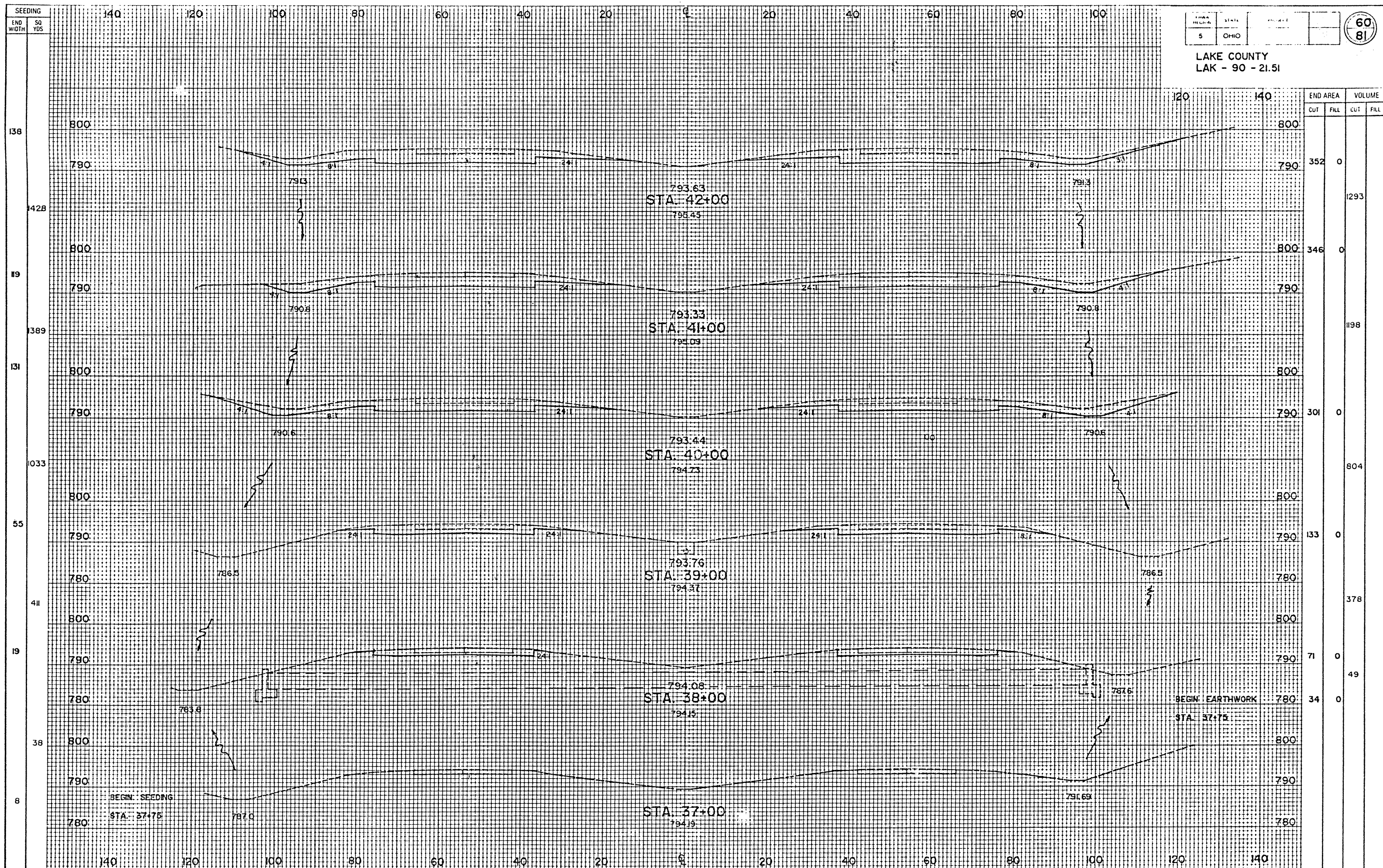
I-90 - STA. 37+00 TO STA. 42+00
