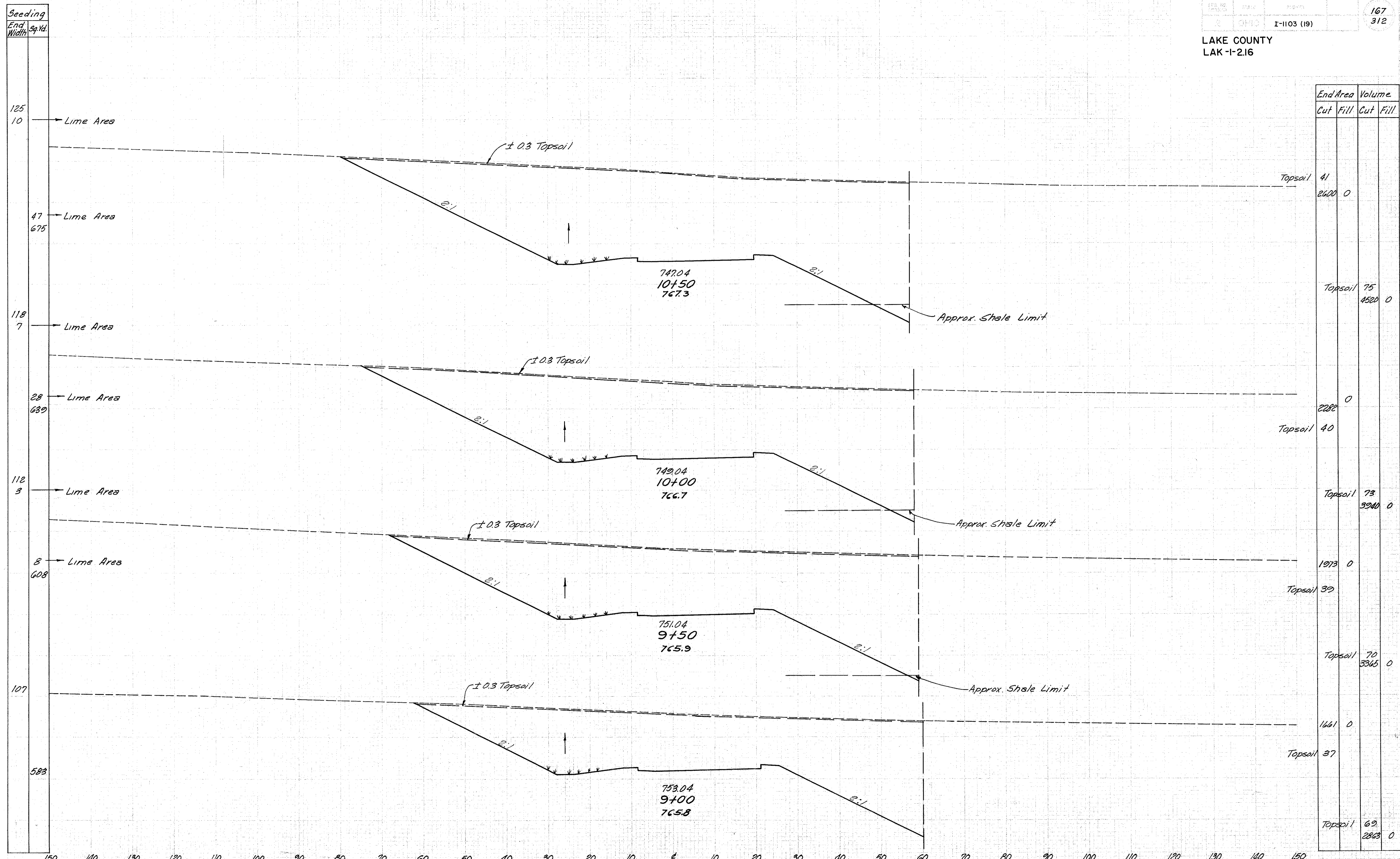
S.R. #91 INTERCHANGE RAMP "B" Sta. 9+00 To Sta. 10+50
