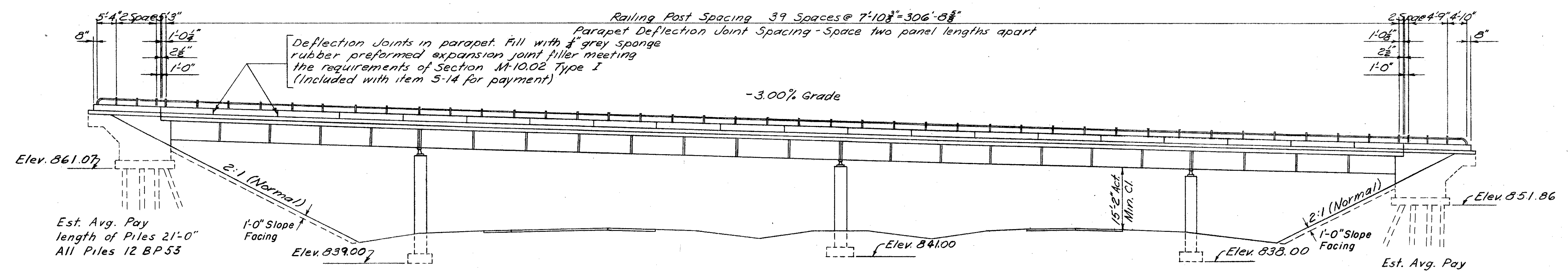
ELEVATION
