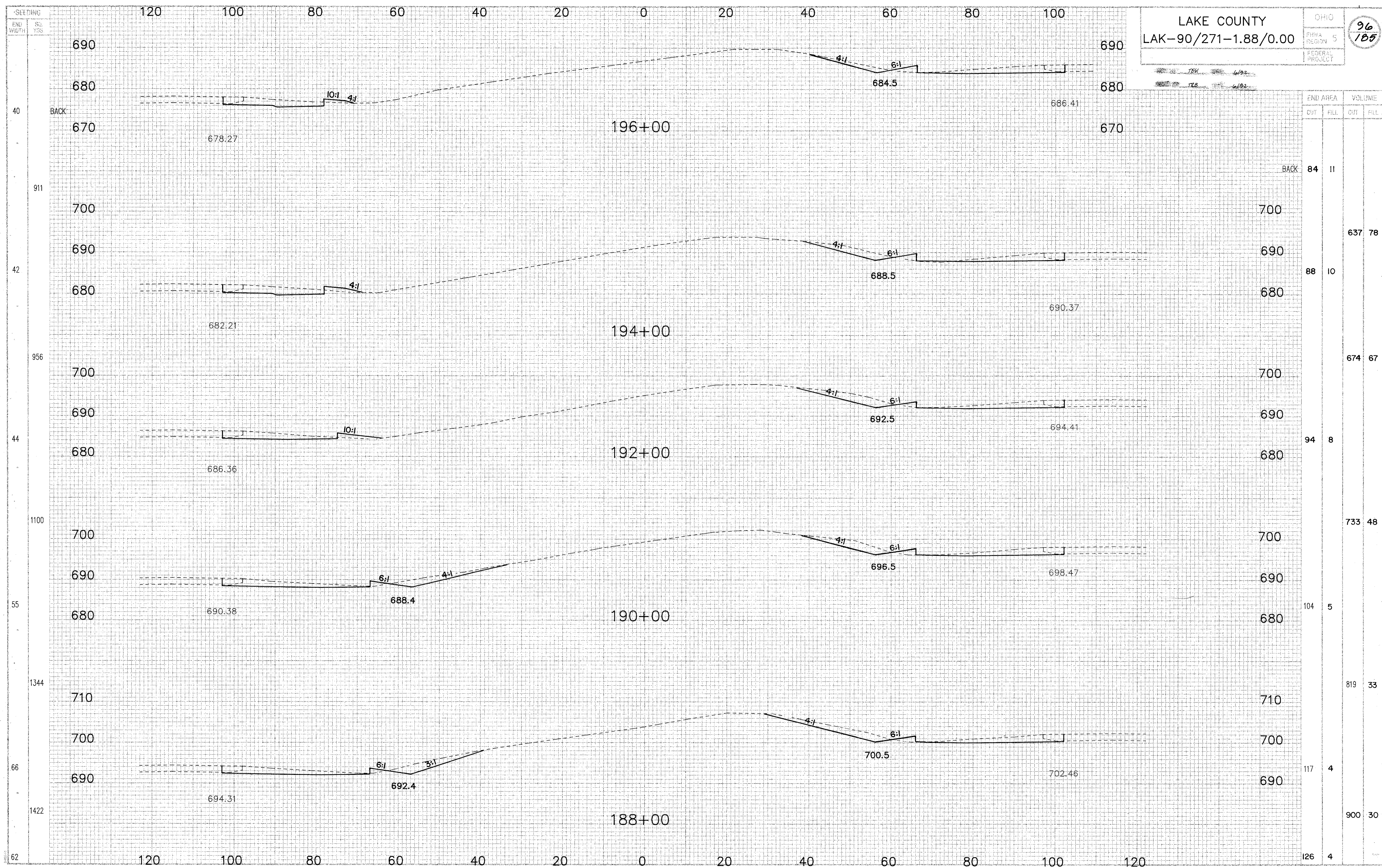
CROSS SECTIONS STA. 188+00 TO STA. 196+00
