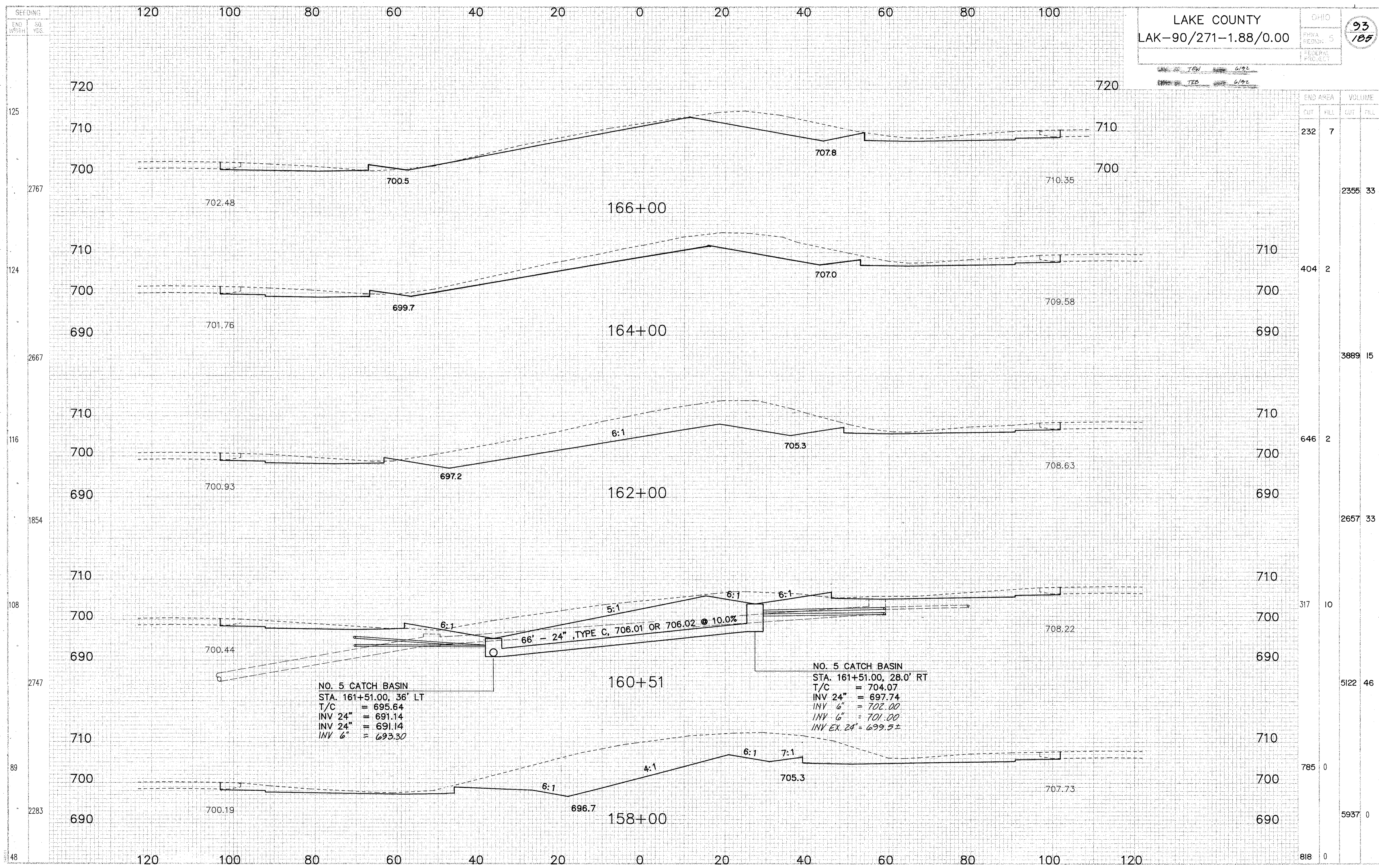
CROSS SECTIONS STA. 158+00 TO STA. 166+00
