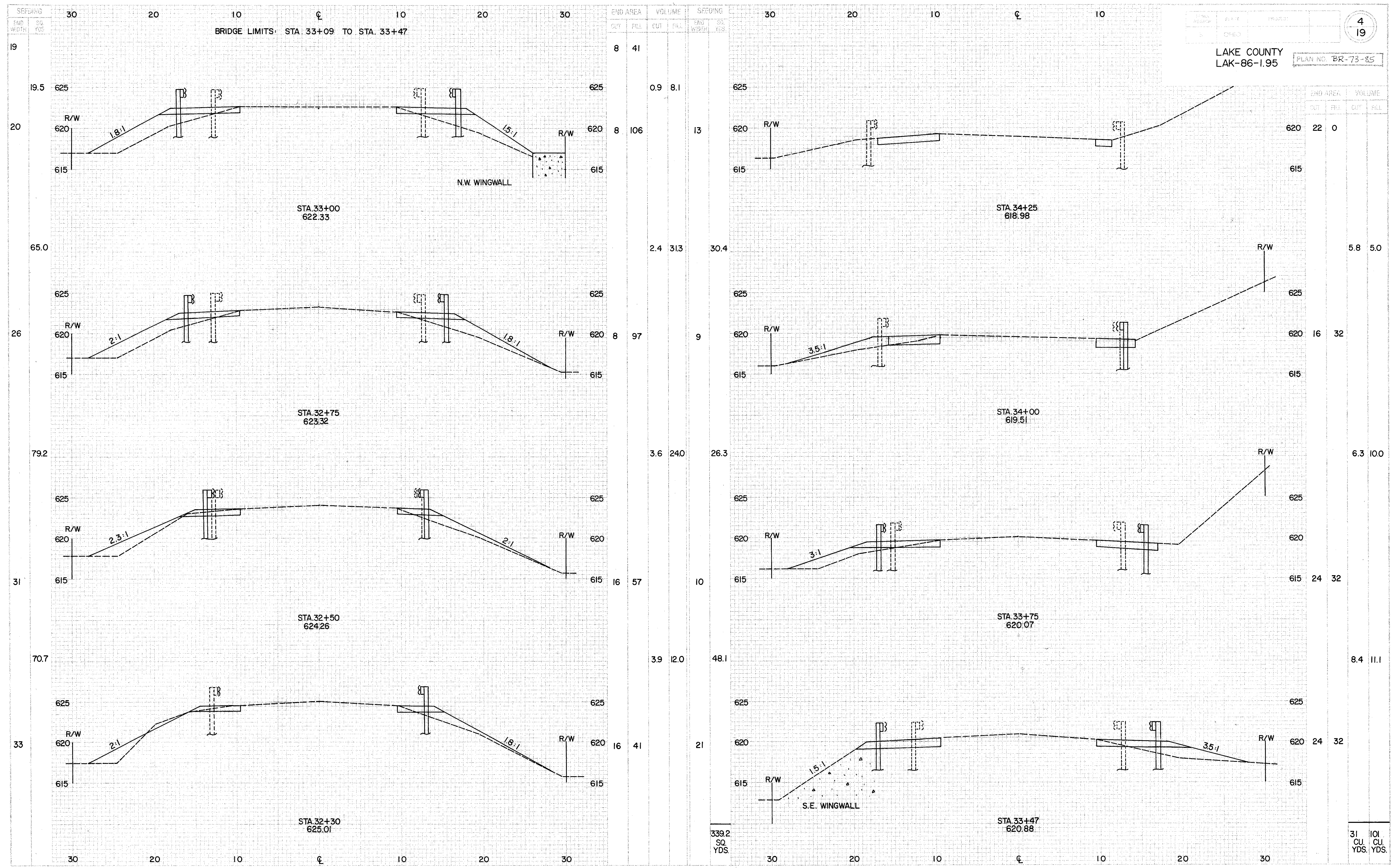
CROSS SECTIONS STA. 32+30 TO STA. 34+25
