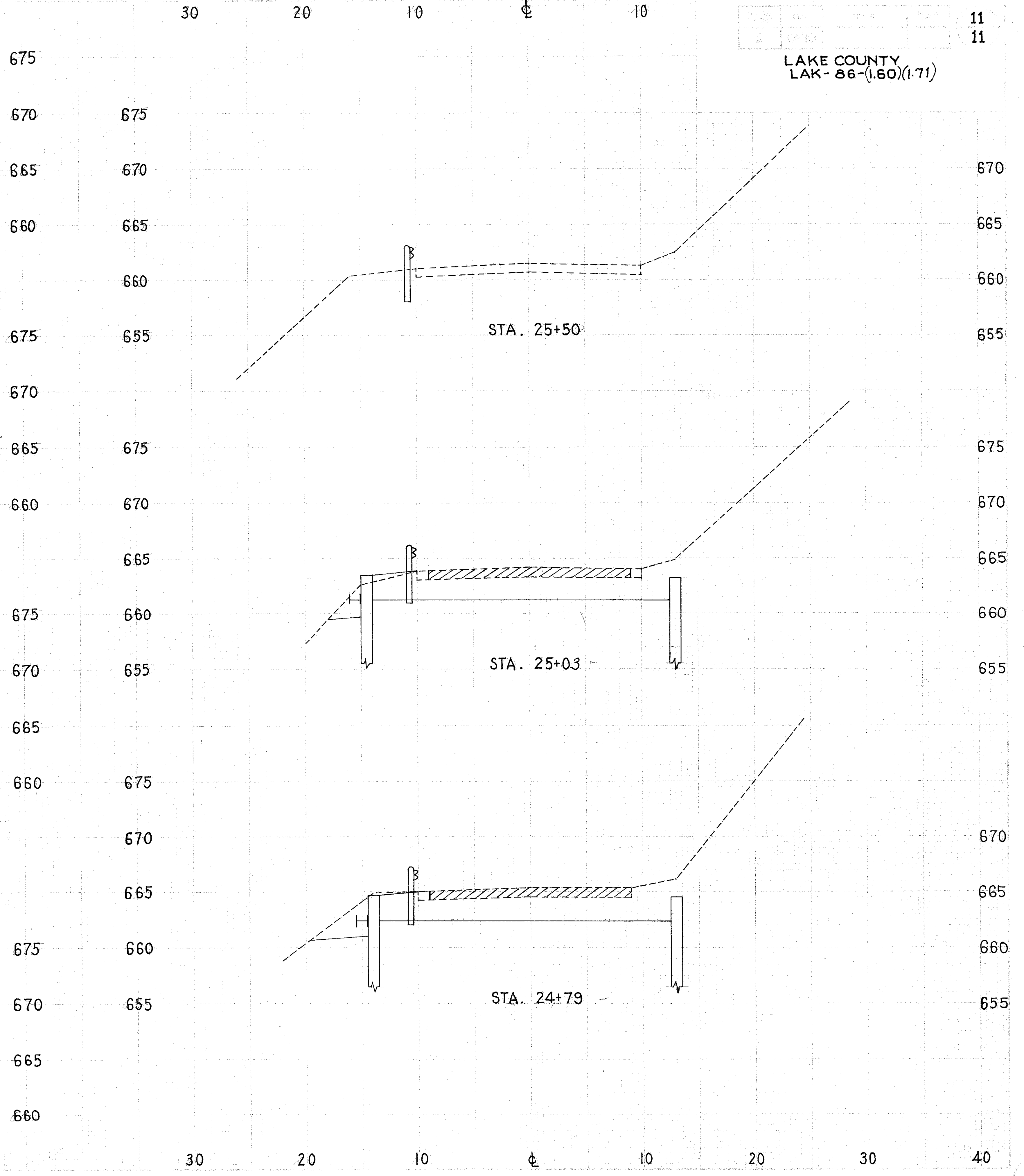
CROSS SECTIONS S.R. 86 STA. 23+50 TO STA. 25+50
