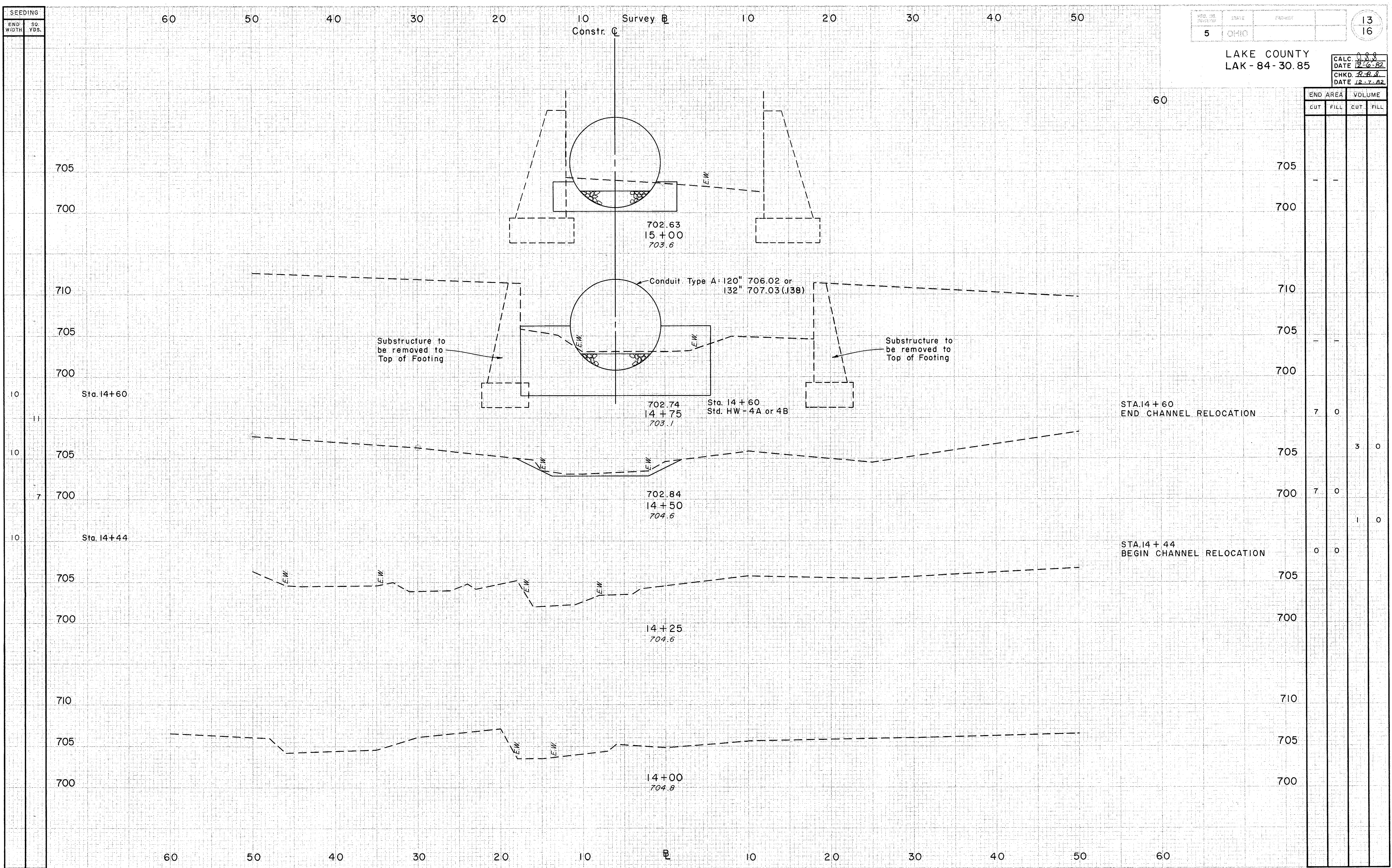
ARCOLA CREEK STA. 14+00 TO STA. 15+00
