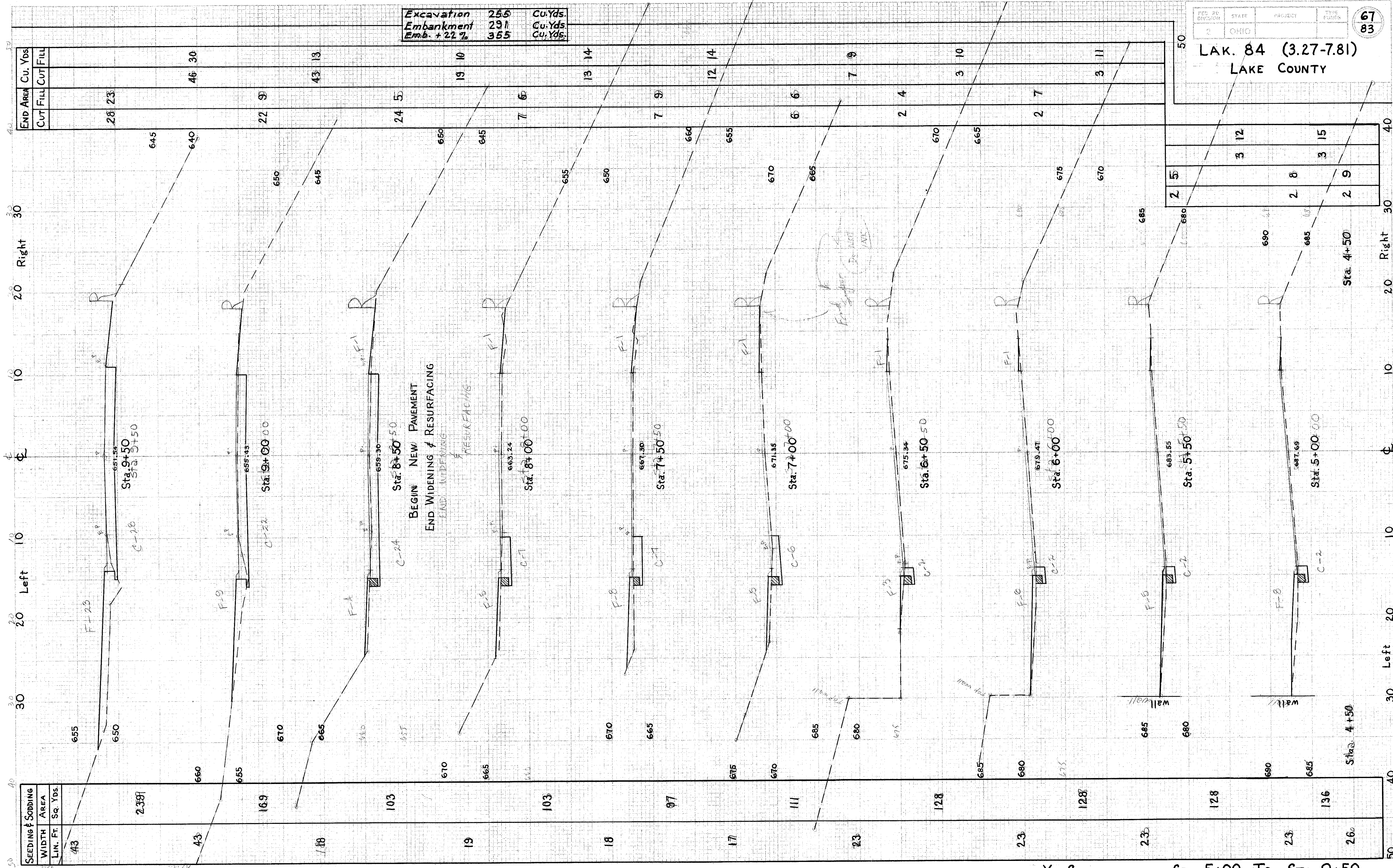
X SECTIONS STA. 5+00 TO STA. 9+50
