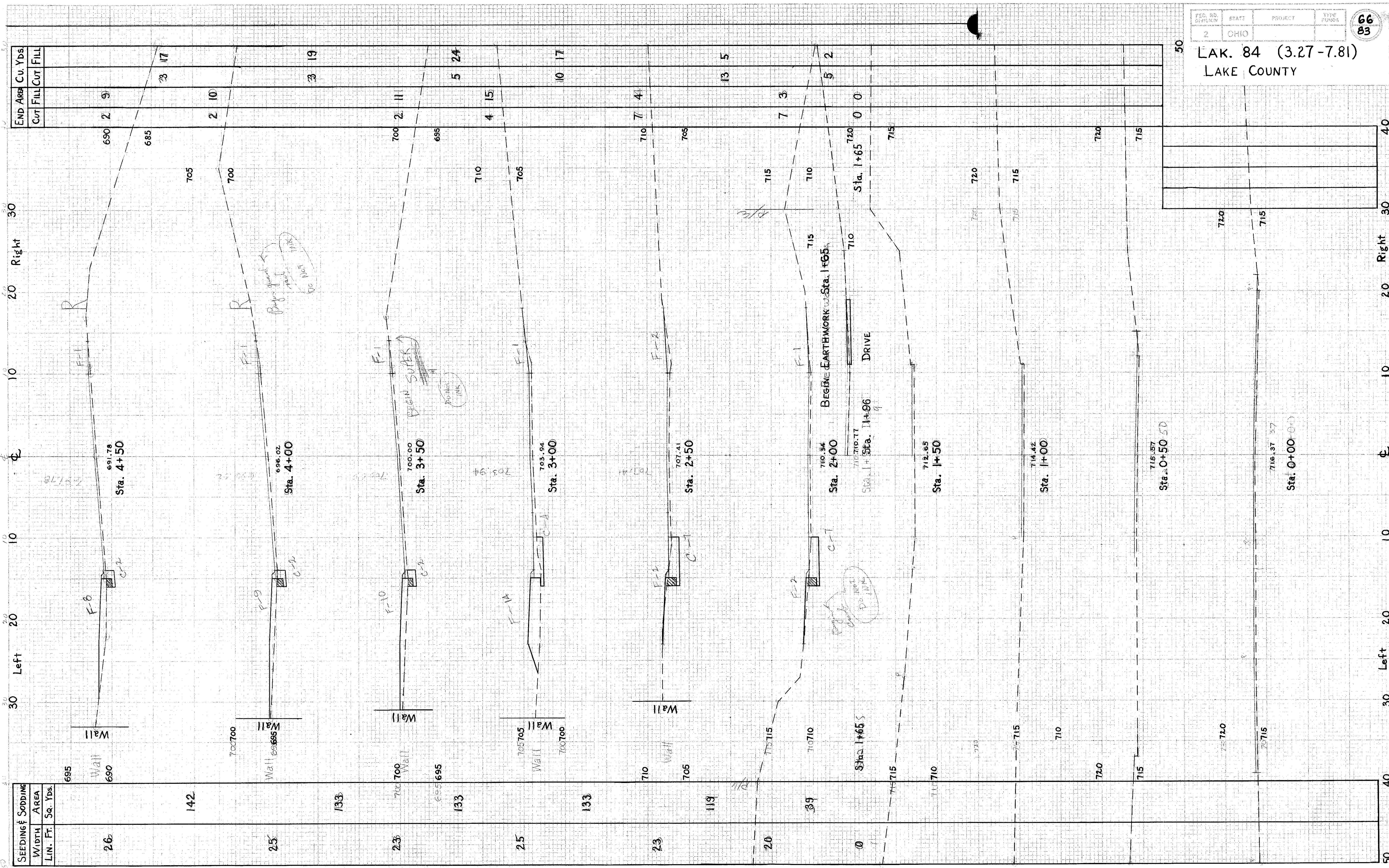
X SECTIONS STA. 0+00 TO STA. 4+50
