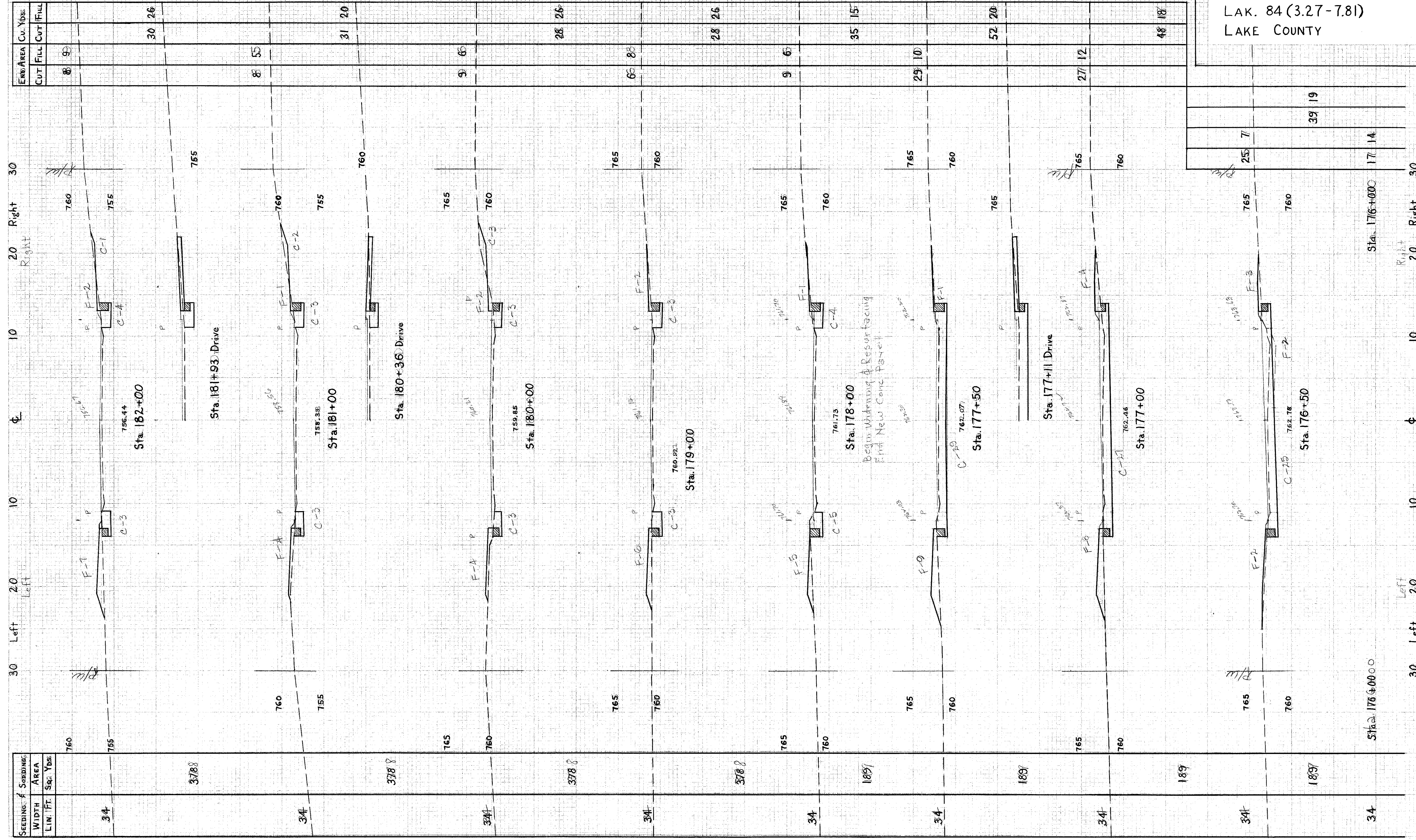
X SECTIONS STA. 176+50 To STA. 182+00
