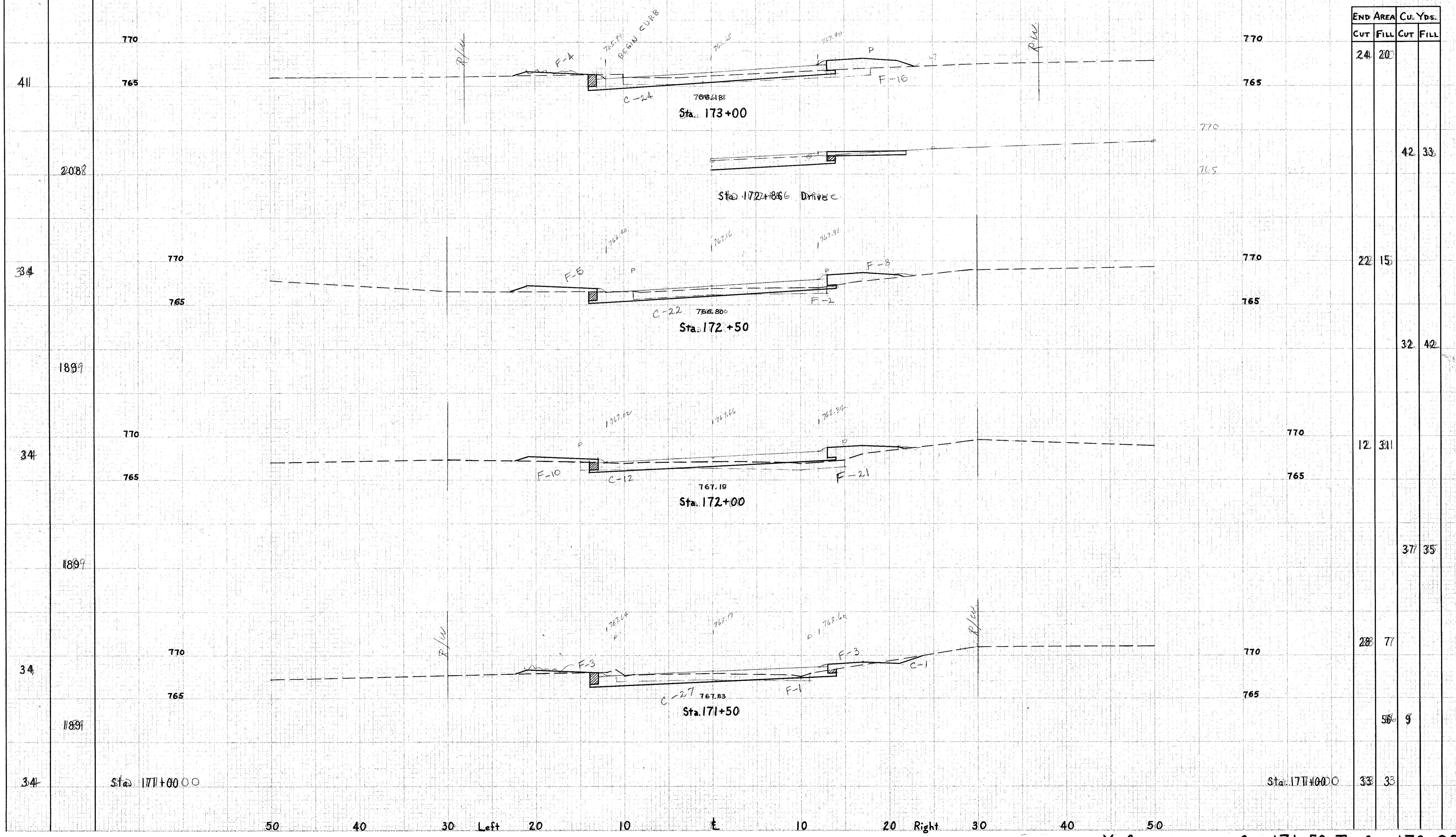
X SECTIONS STA. 171+50 TO STA. 173+00
