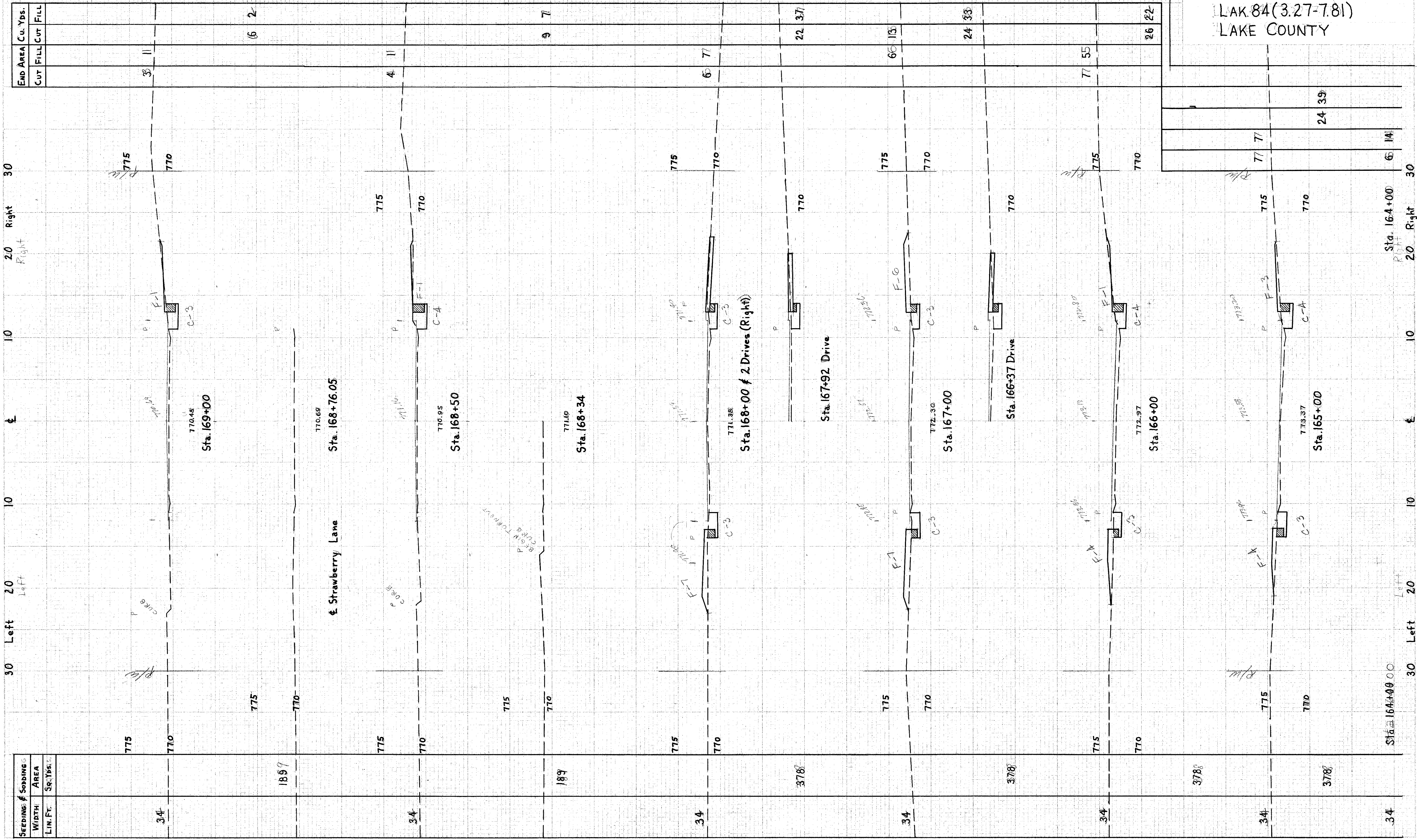
X SECTIONS STA. 165+00 TO STA. 169+00
