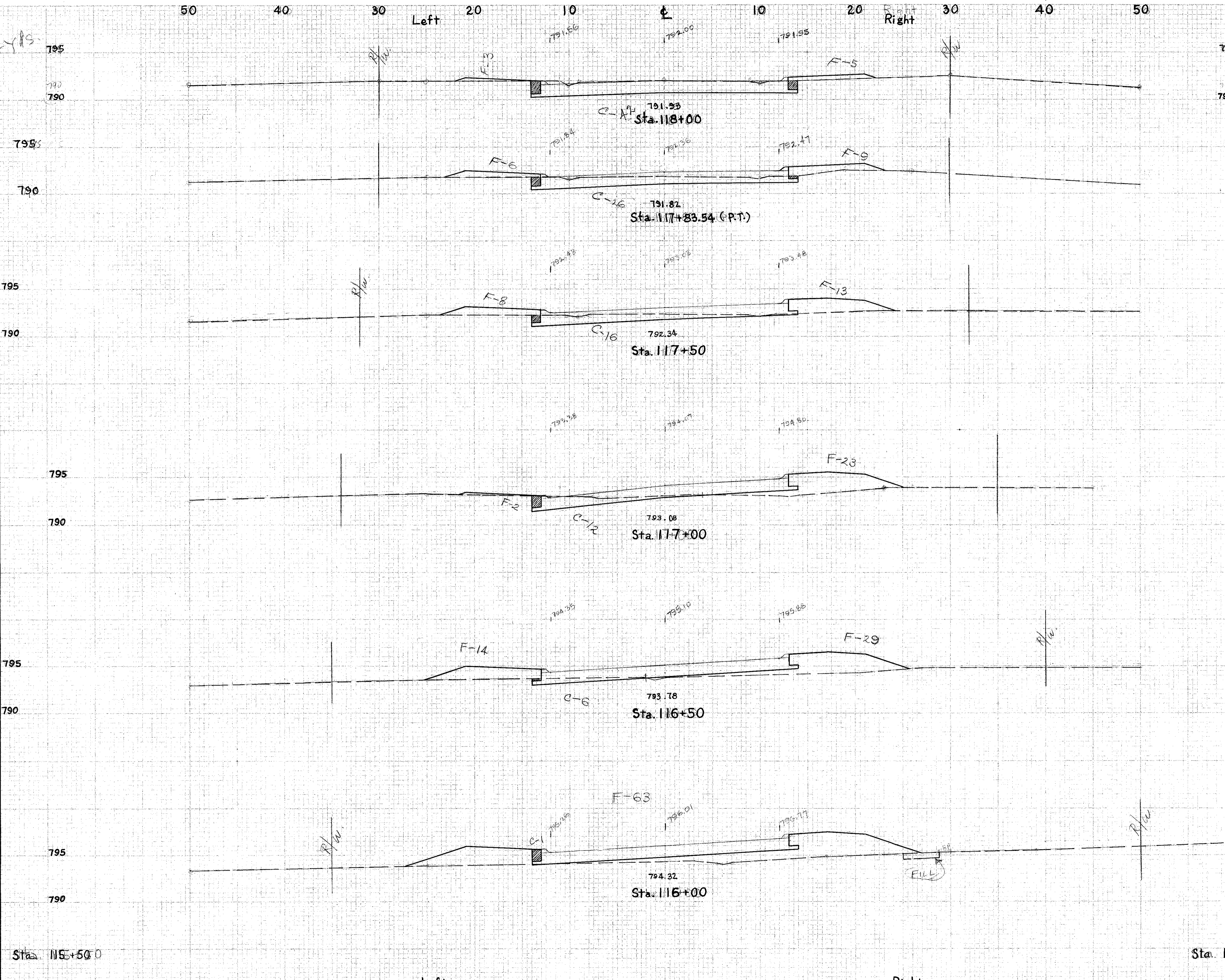
X SECTIONS STA. 116+00 TO STA. 118+00
