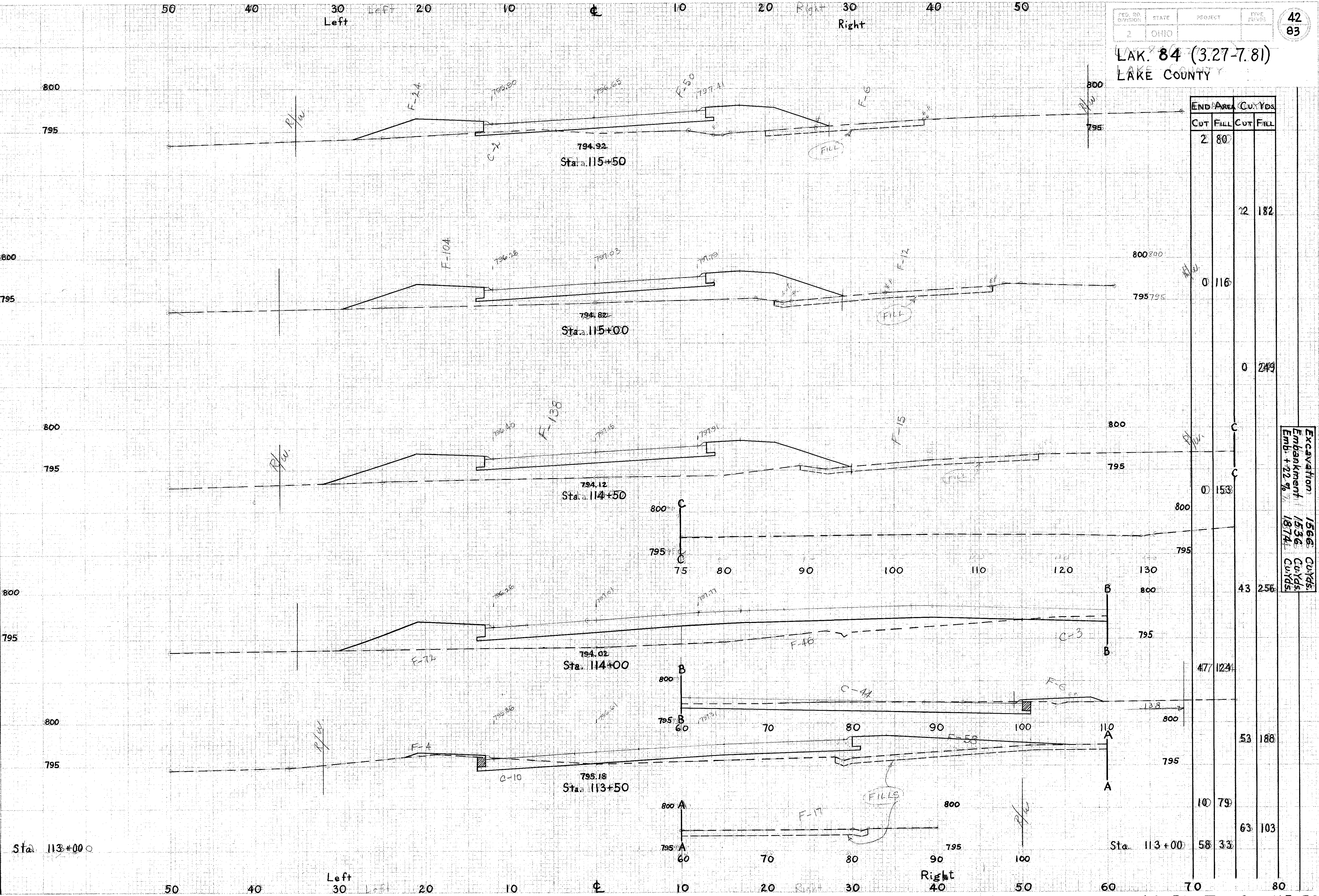
X SECTIONS STA. 113+50 To STA. 115+50
