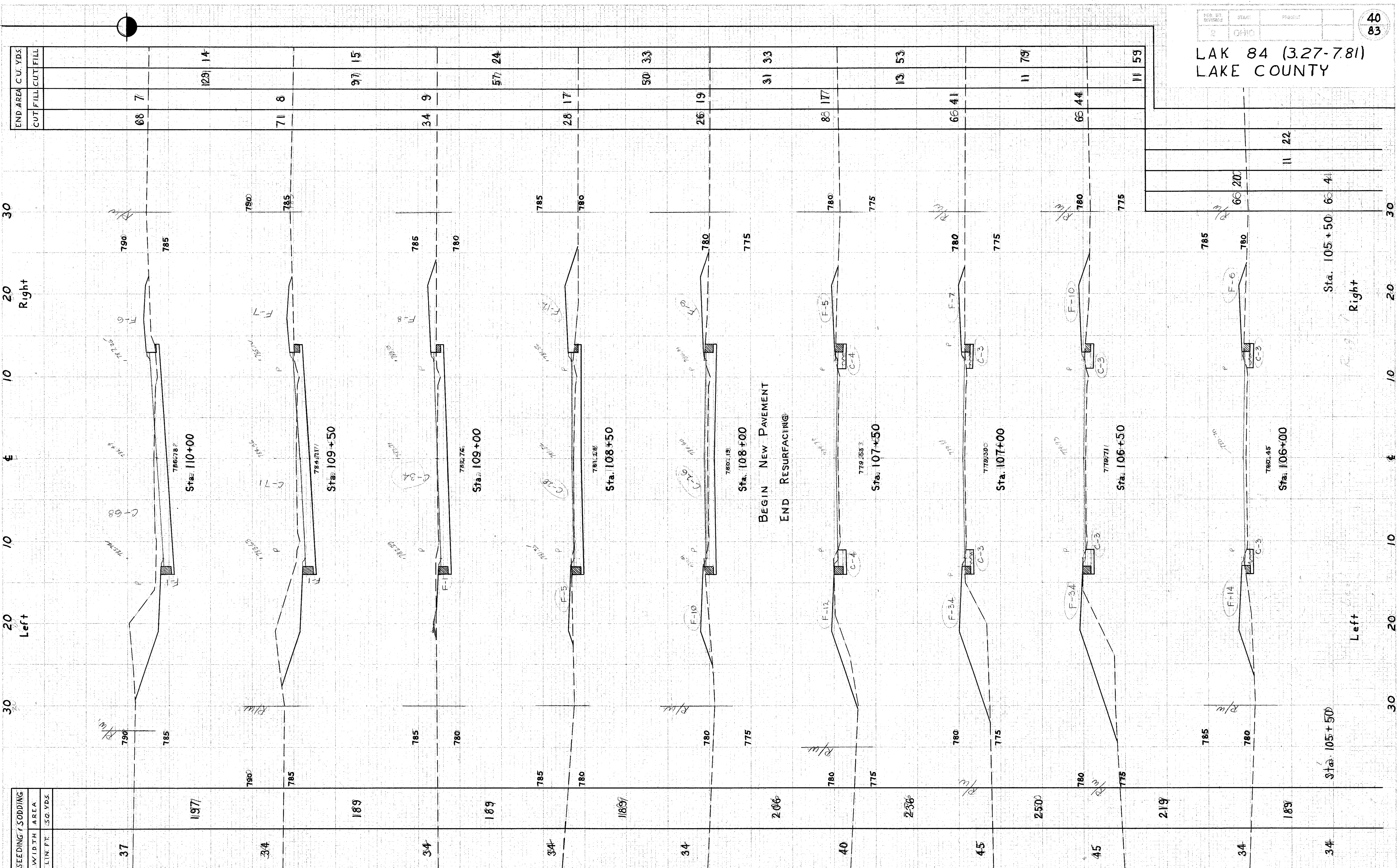
X- Sections Sta. 106+00 To Sta. 110+00
