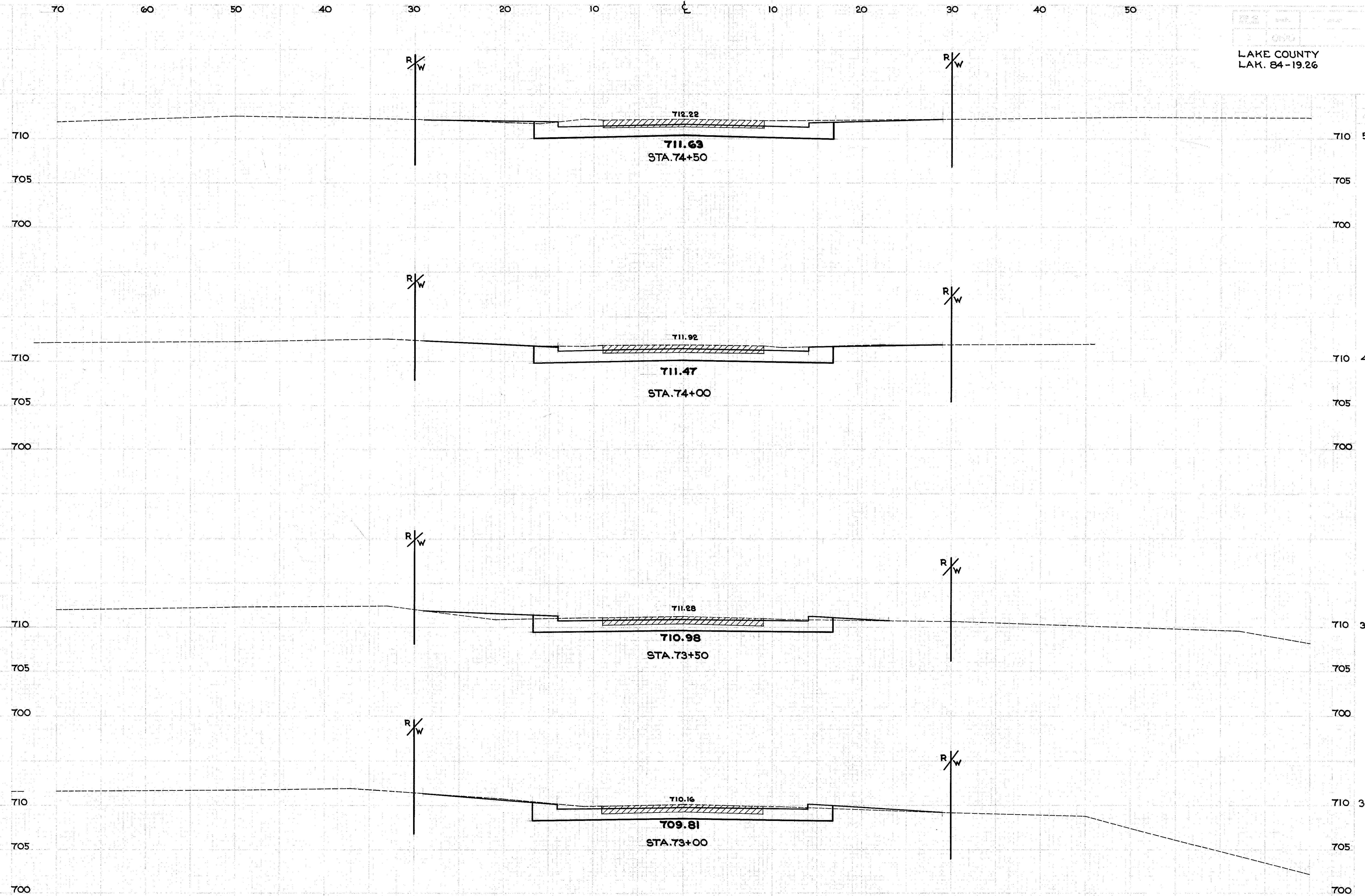
CROSS SECTIONS... S.R. 84... STA. 73+00 to STA. 74+50
