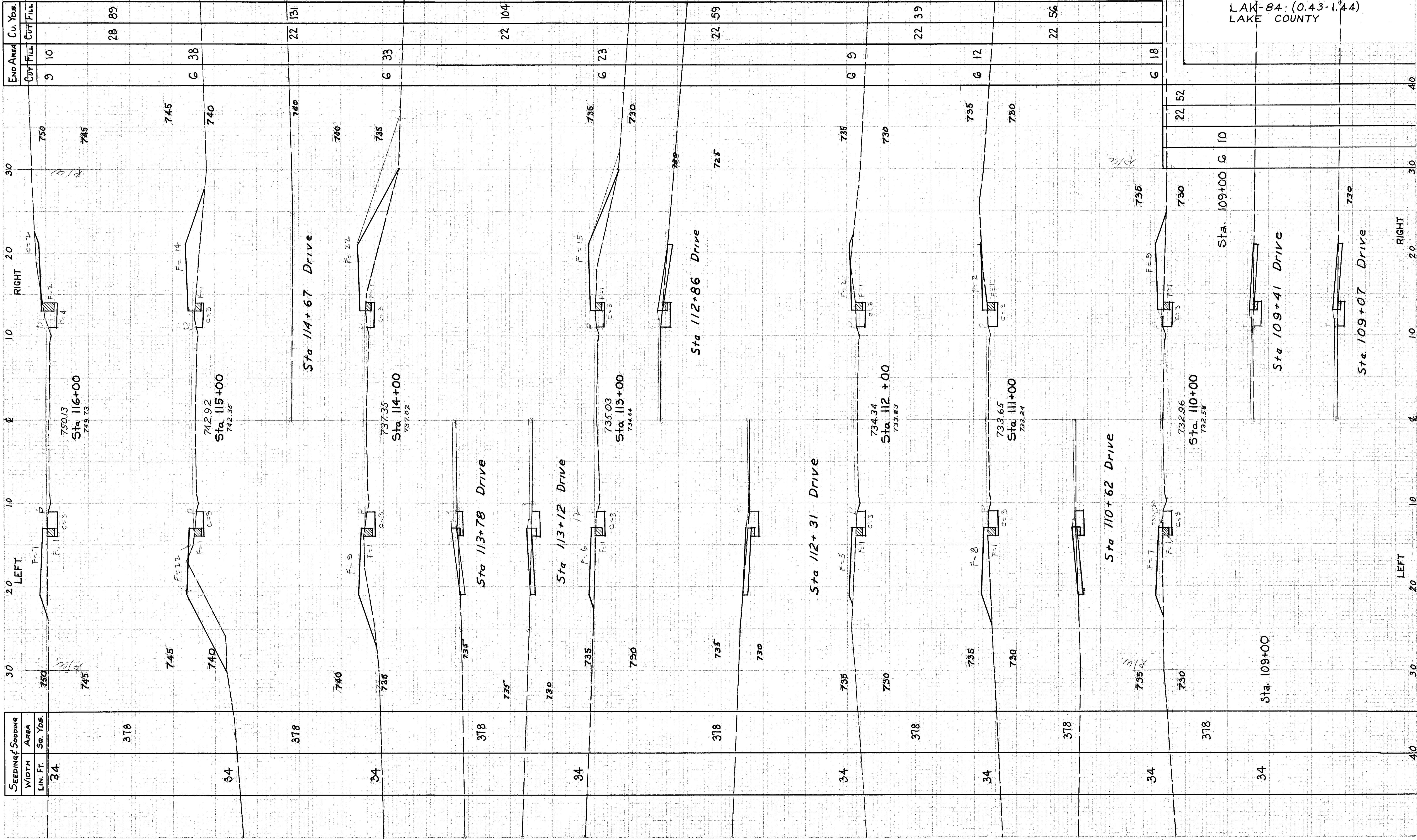
X-SECTIONS STA. 109+07 TO STA. 116+00
