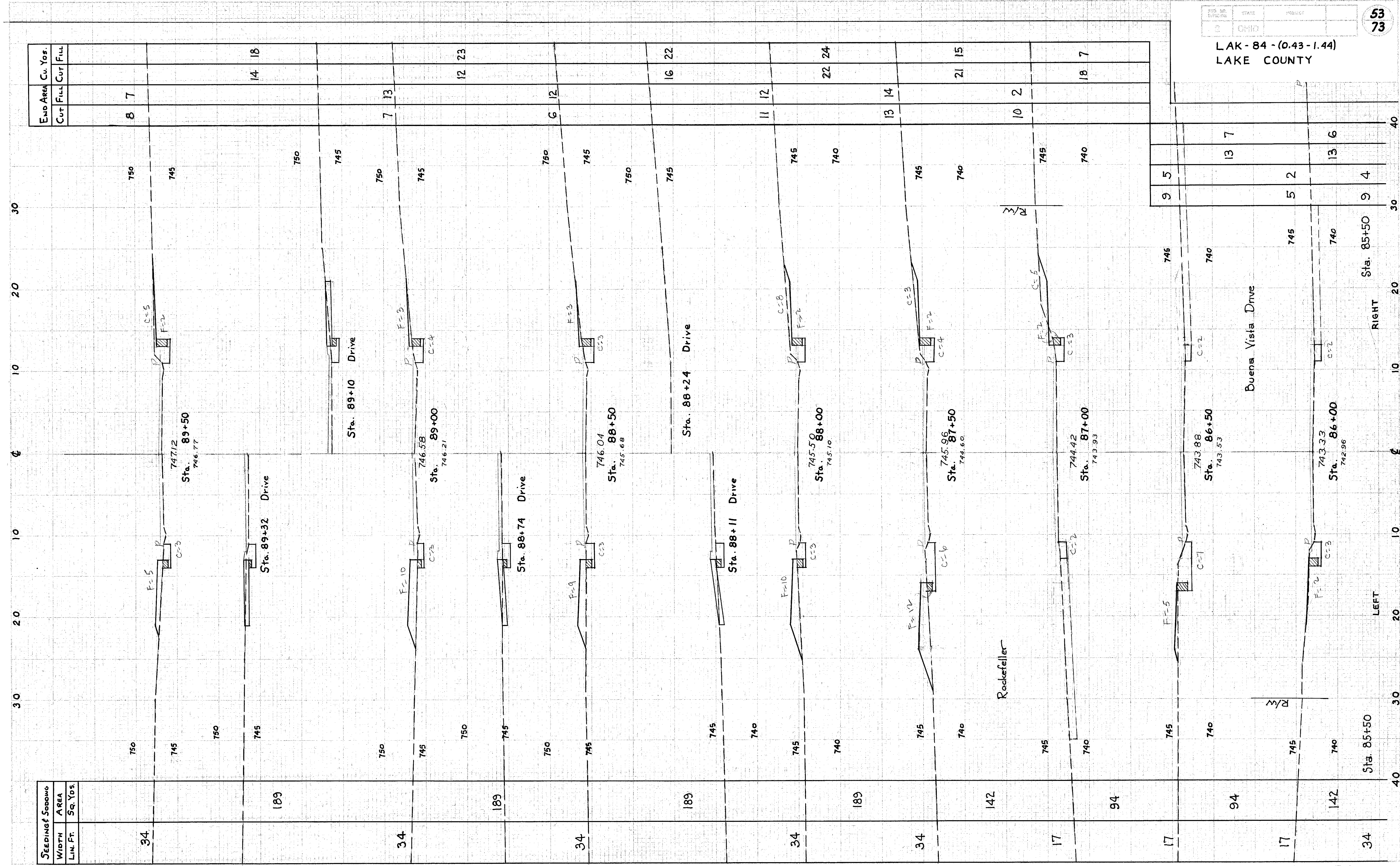
X-SECTIONS STA. 86+00 TO STA. 89+50
