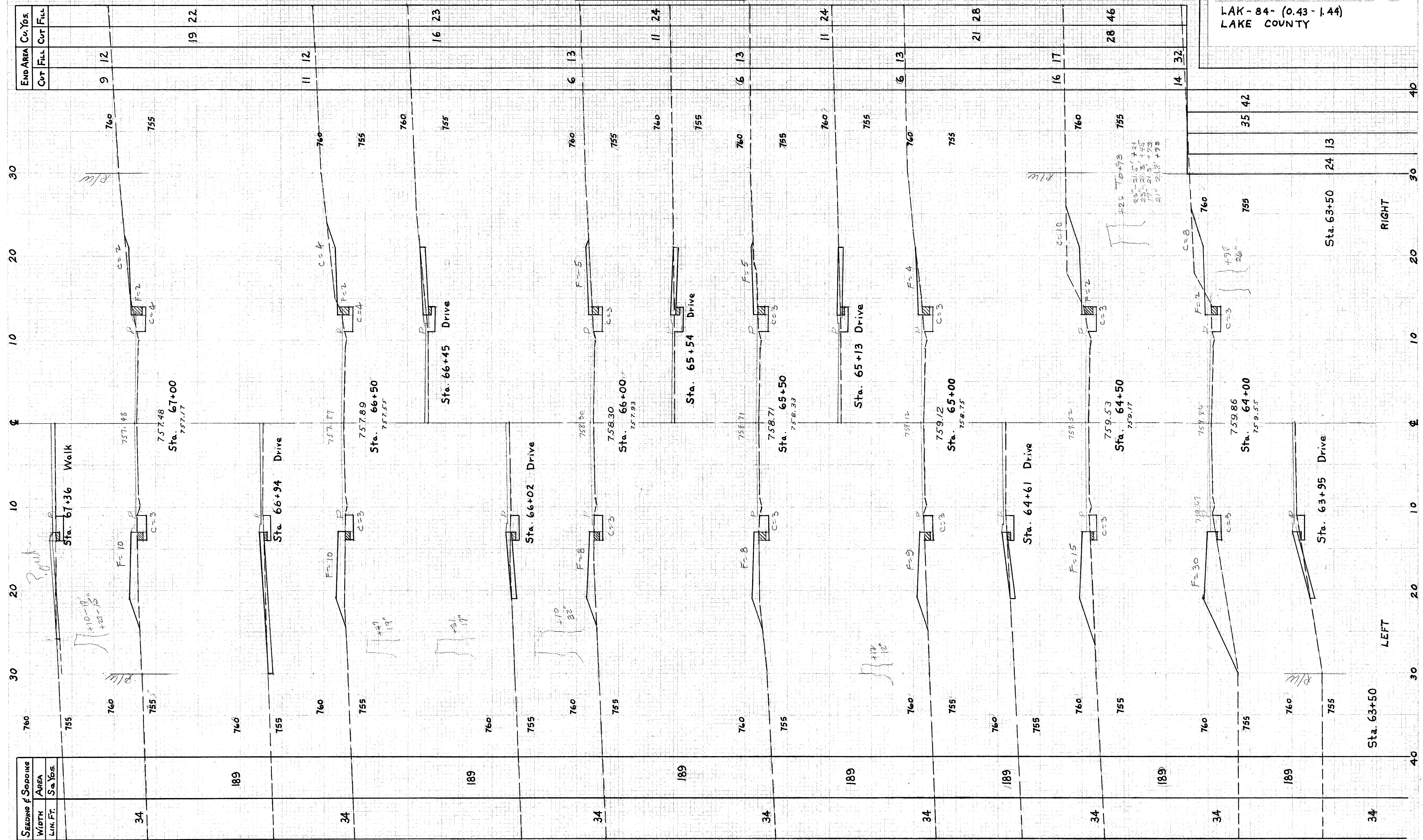
X-SECTIONS STA. 63+95 TO STA. 67+36
