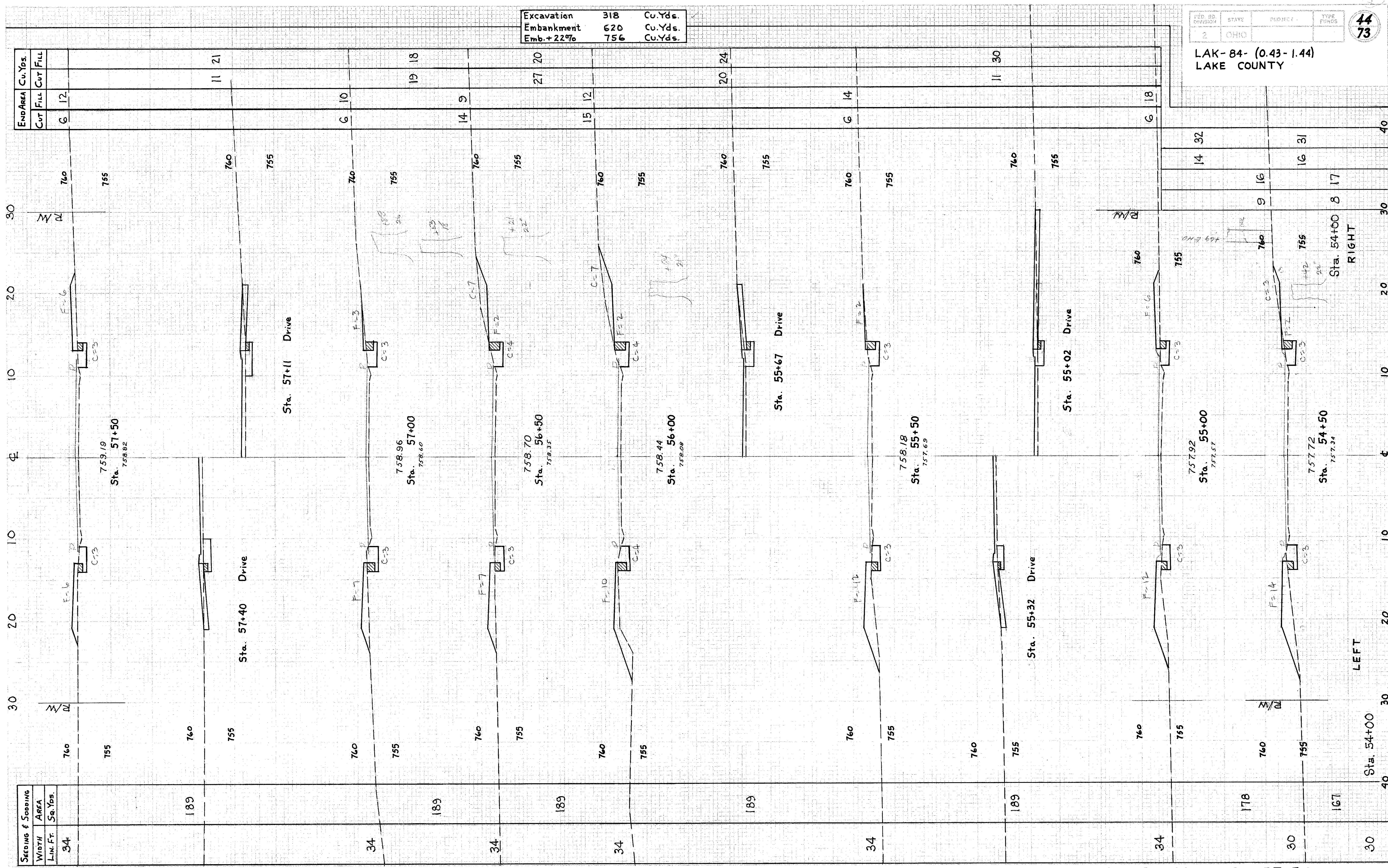
X-SECTIONS STA. 54+50 TO STA. 57+50
