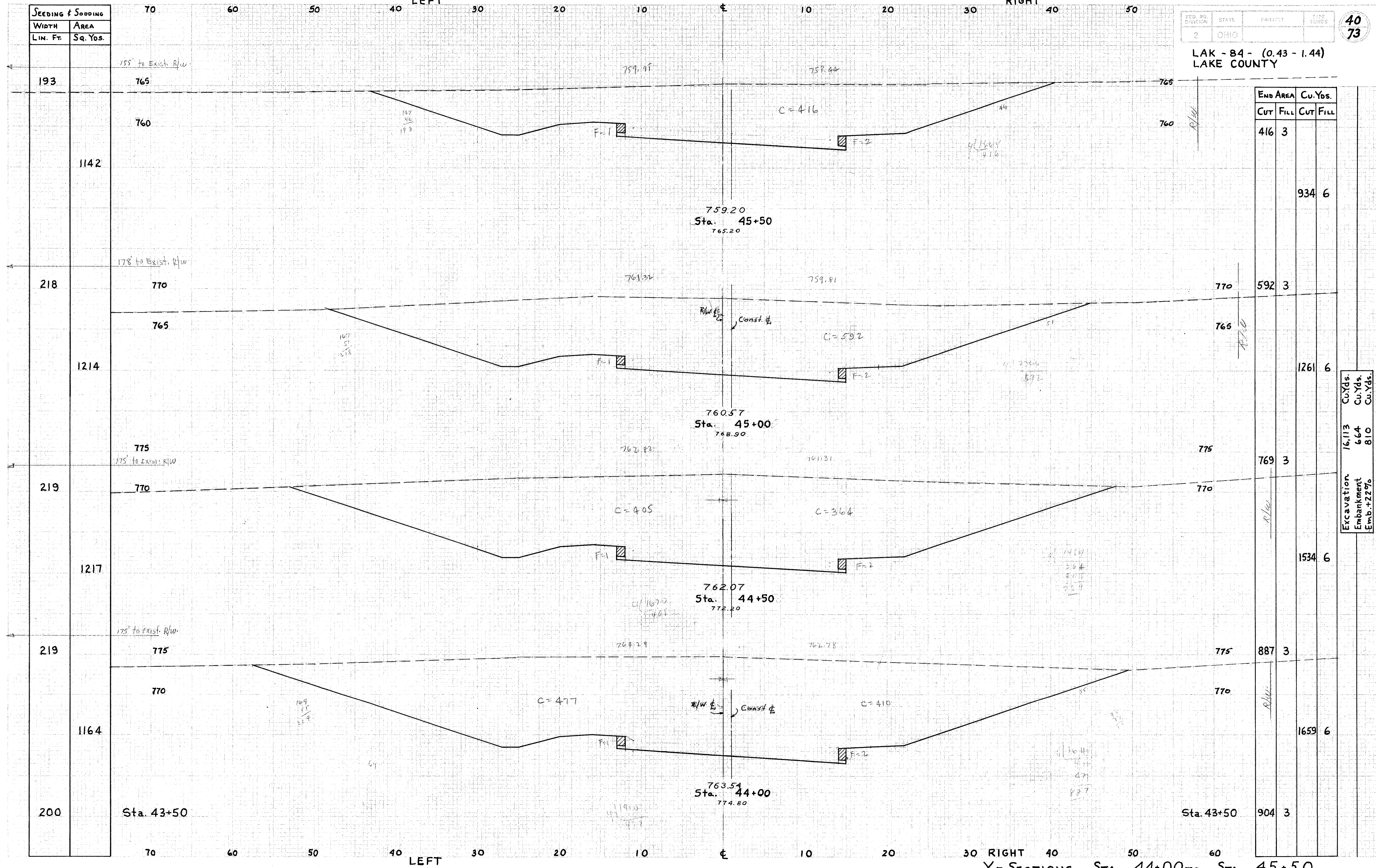
X-SECTIONS STA. 44+00 TO STA. 45+50
