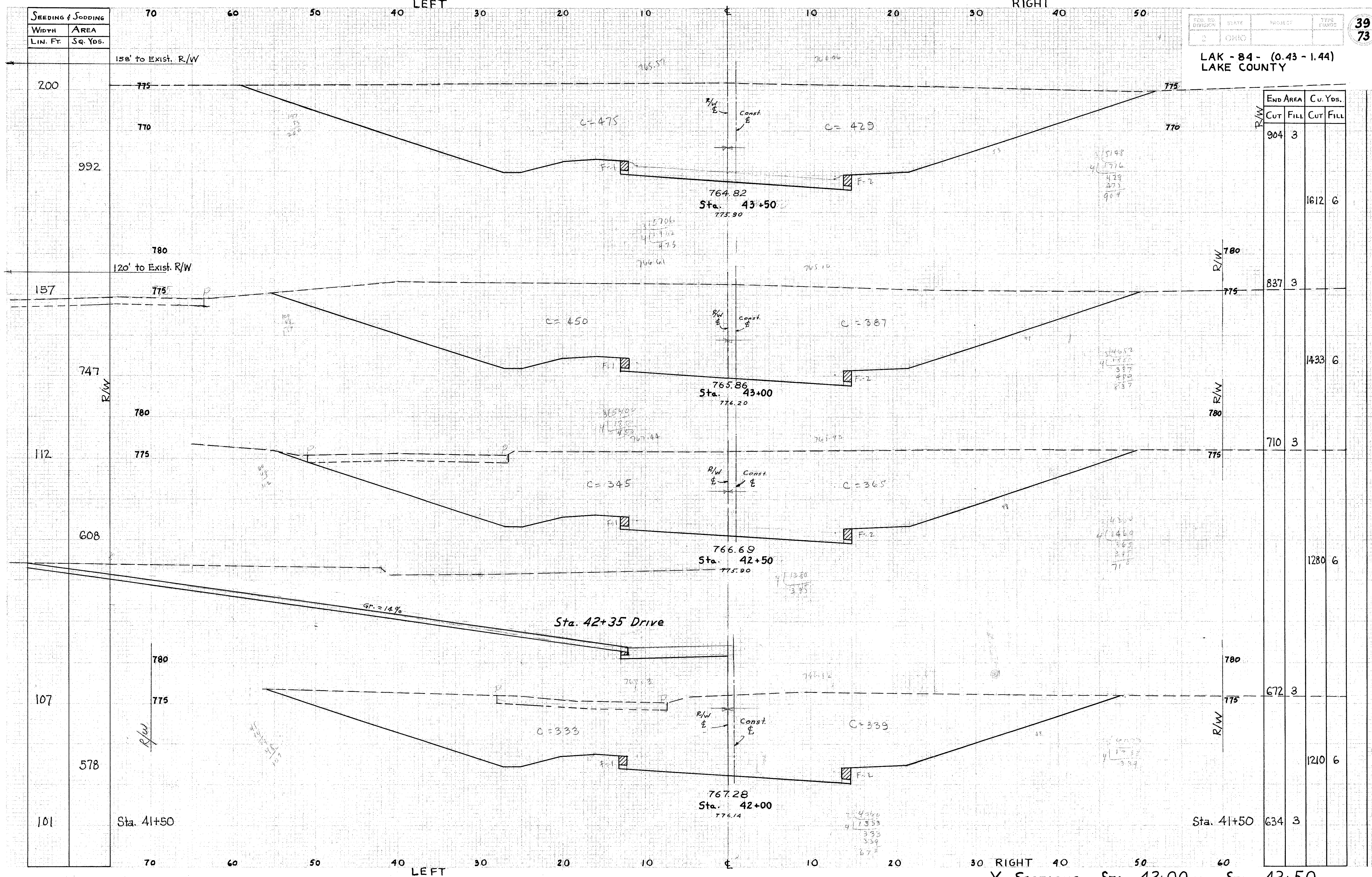
X-SECTIONS STA. 42+00 TO STA. 43+50
