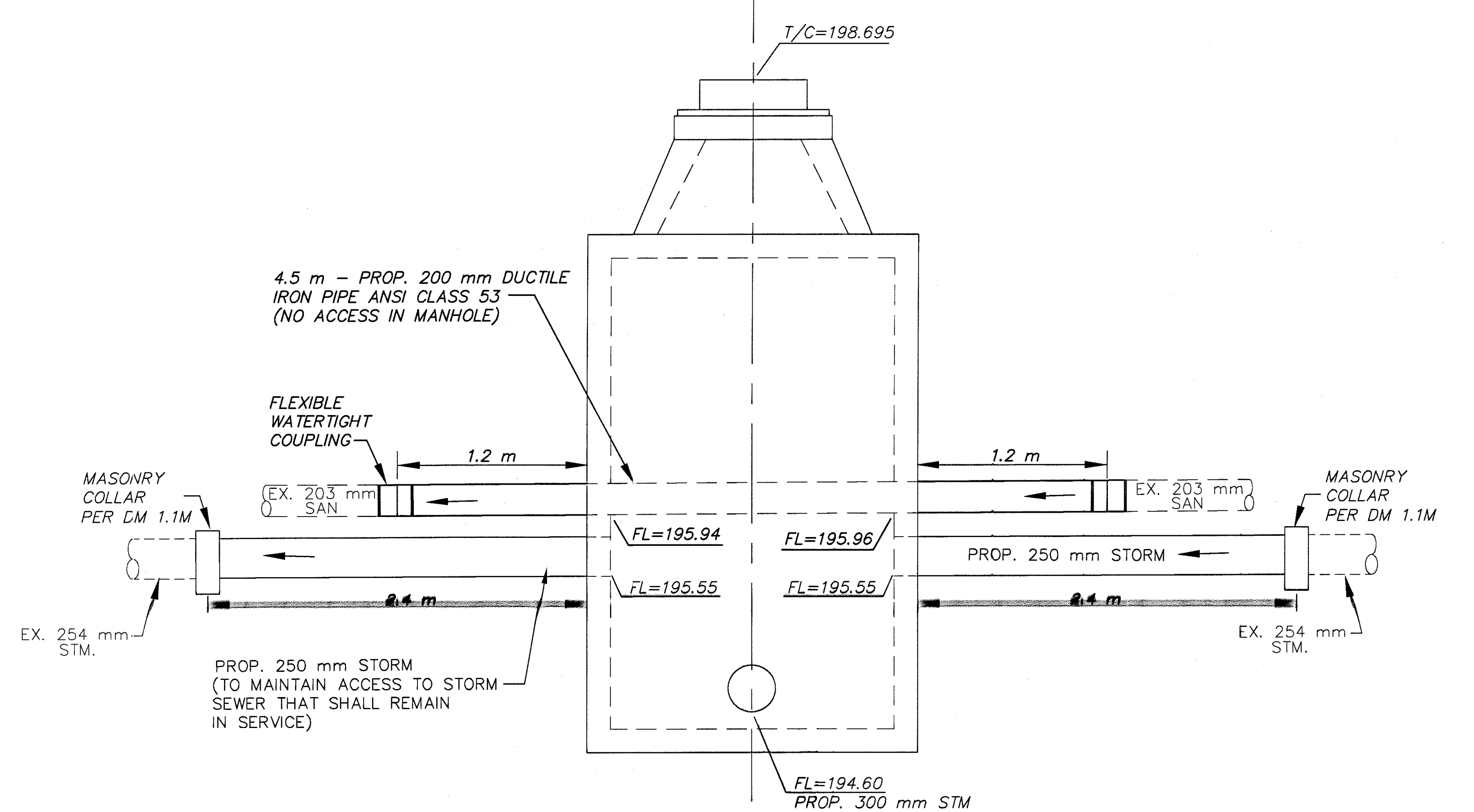
SECTION A-A STA. 5+375.0, C
