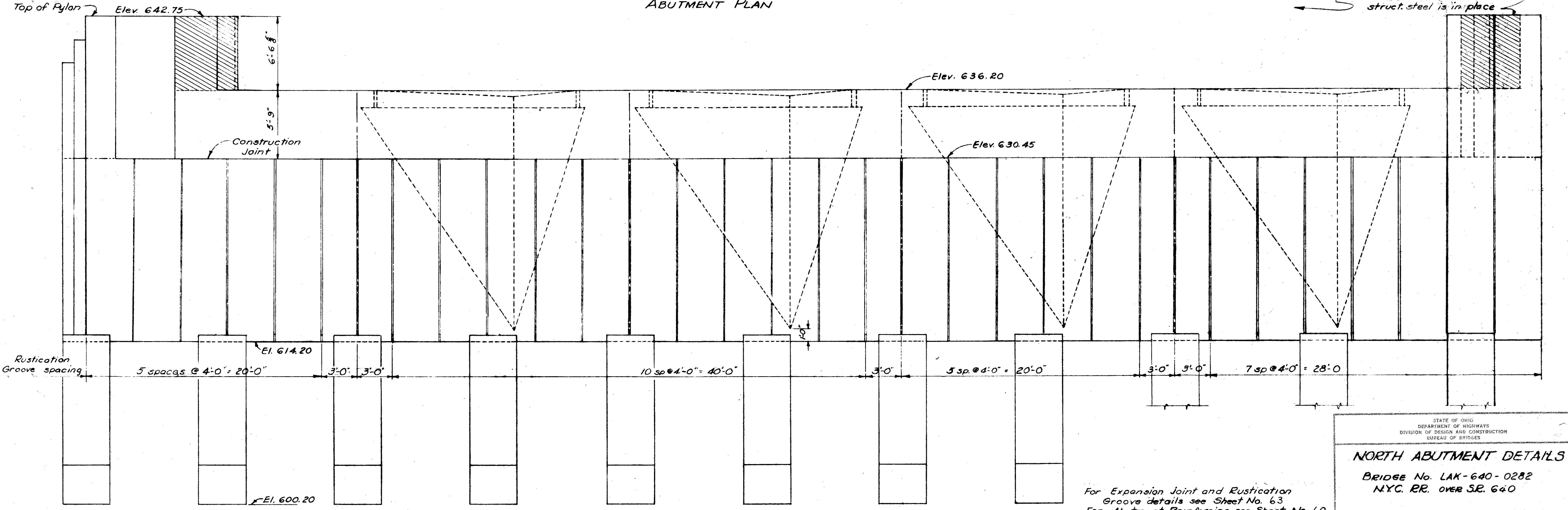
ELEVATION
