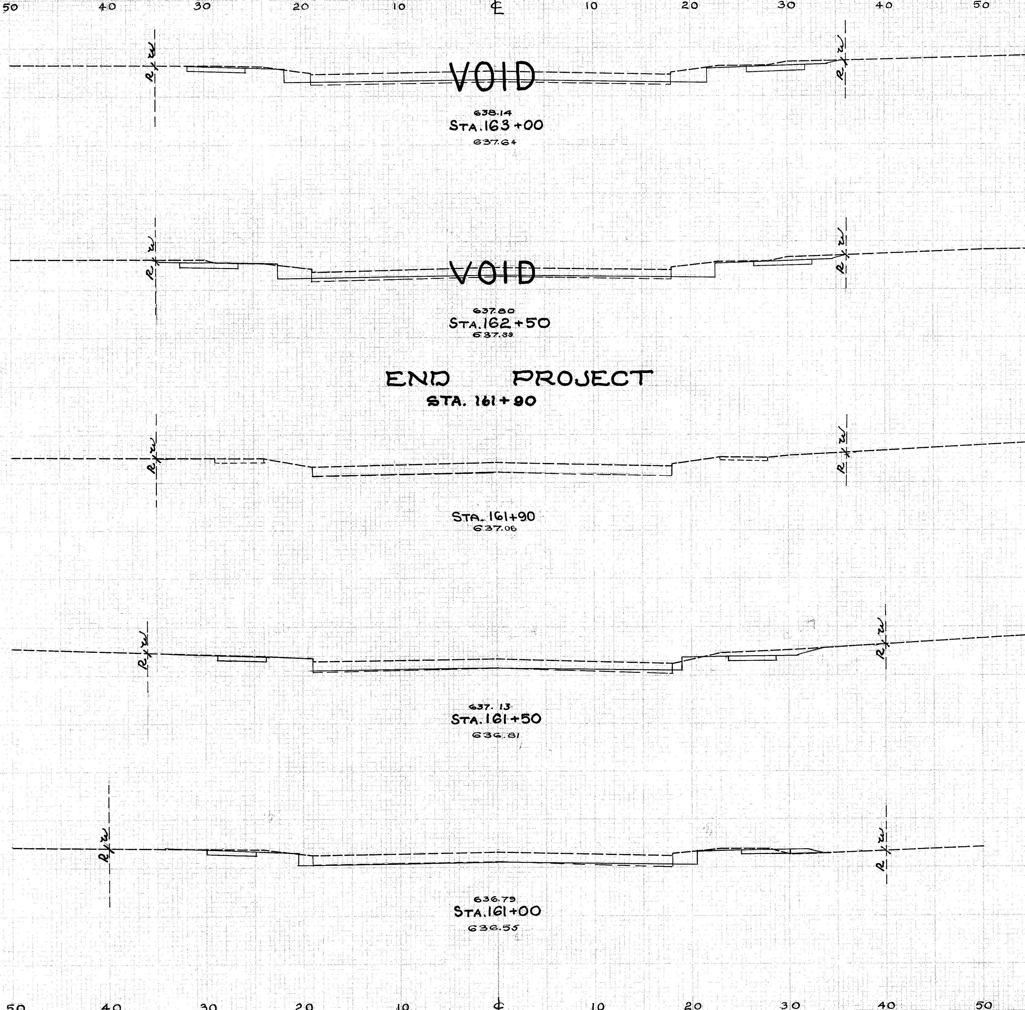
X-SECTIONS STA. 161+00 TO STA. 163+00
