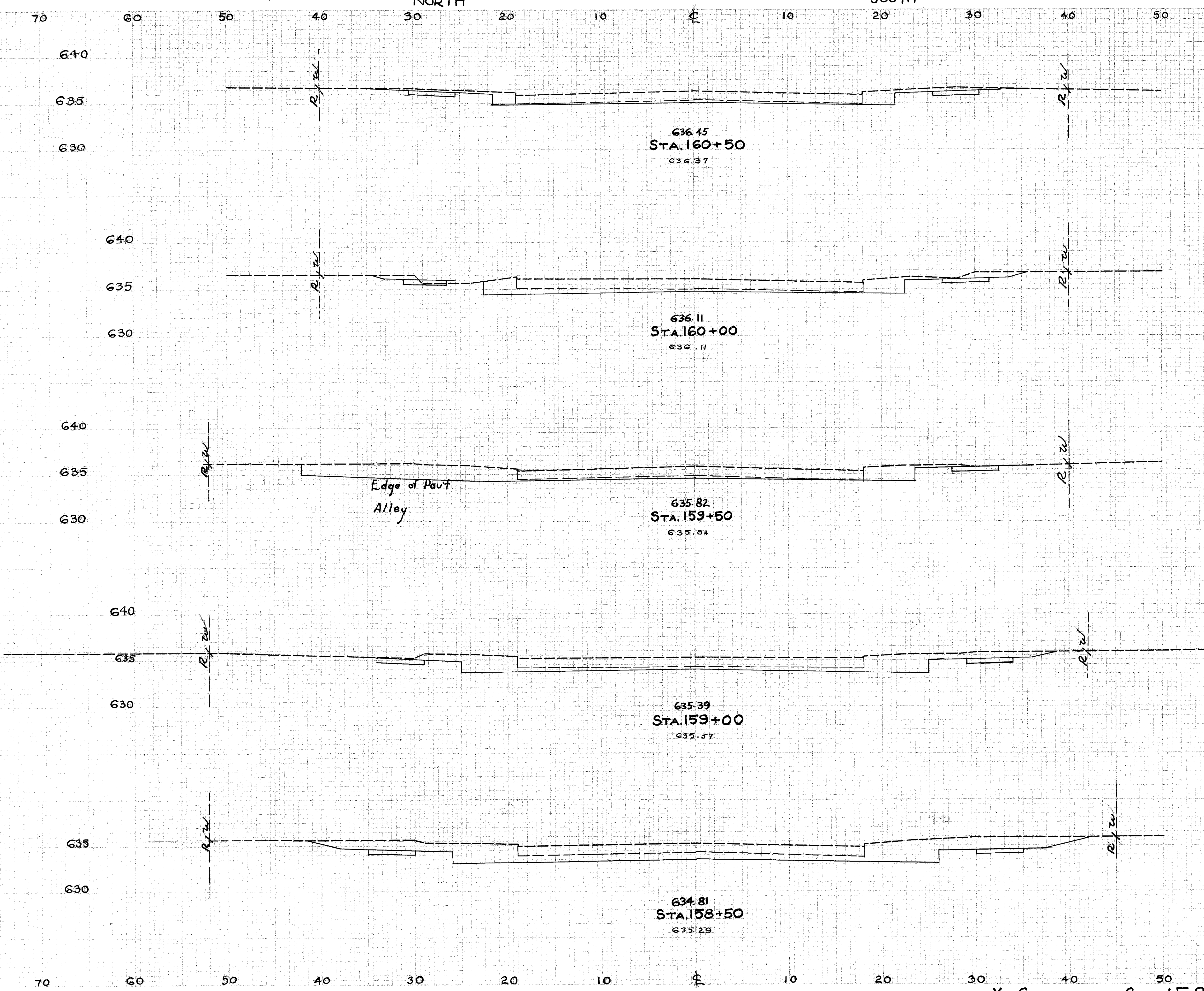
X-SECTIONS STA. 158+50 TO STA. 160+50
