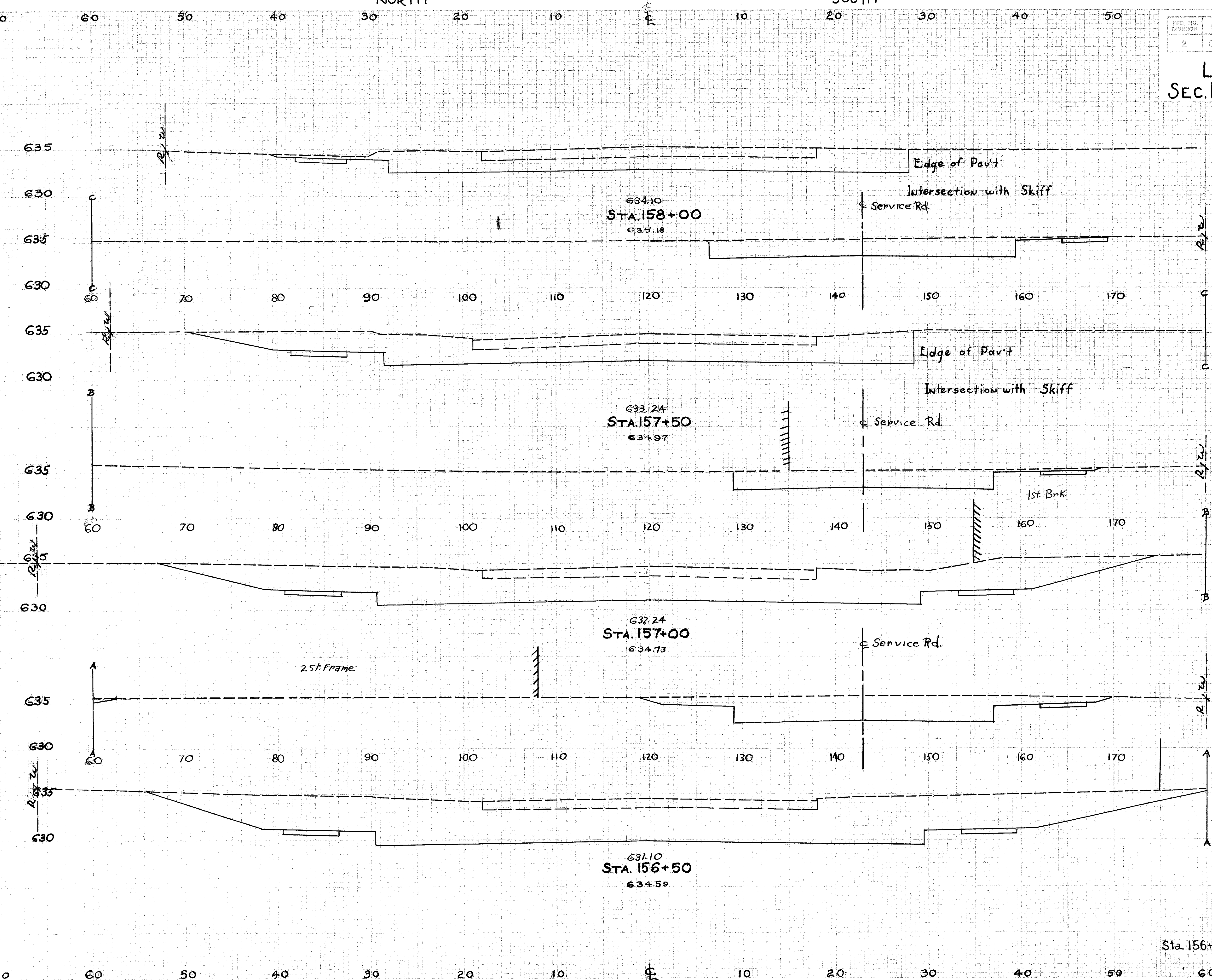
X-SECTIONS STA. 156+50 TO STA. 158+00
