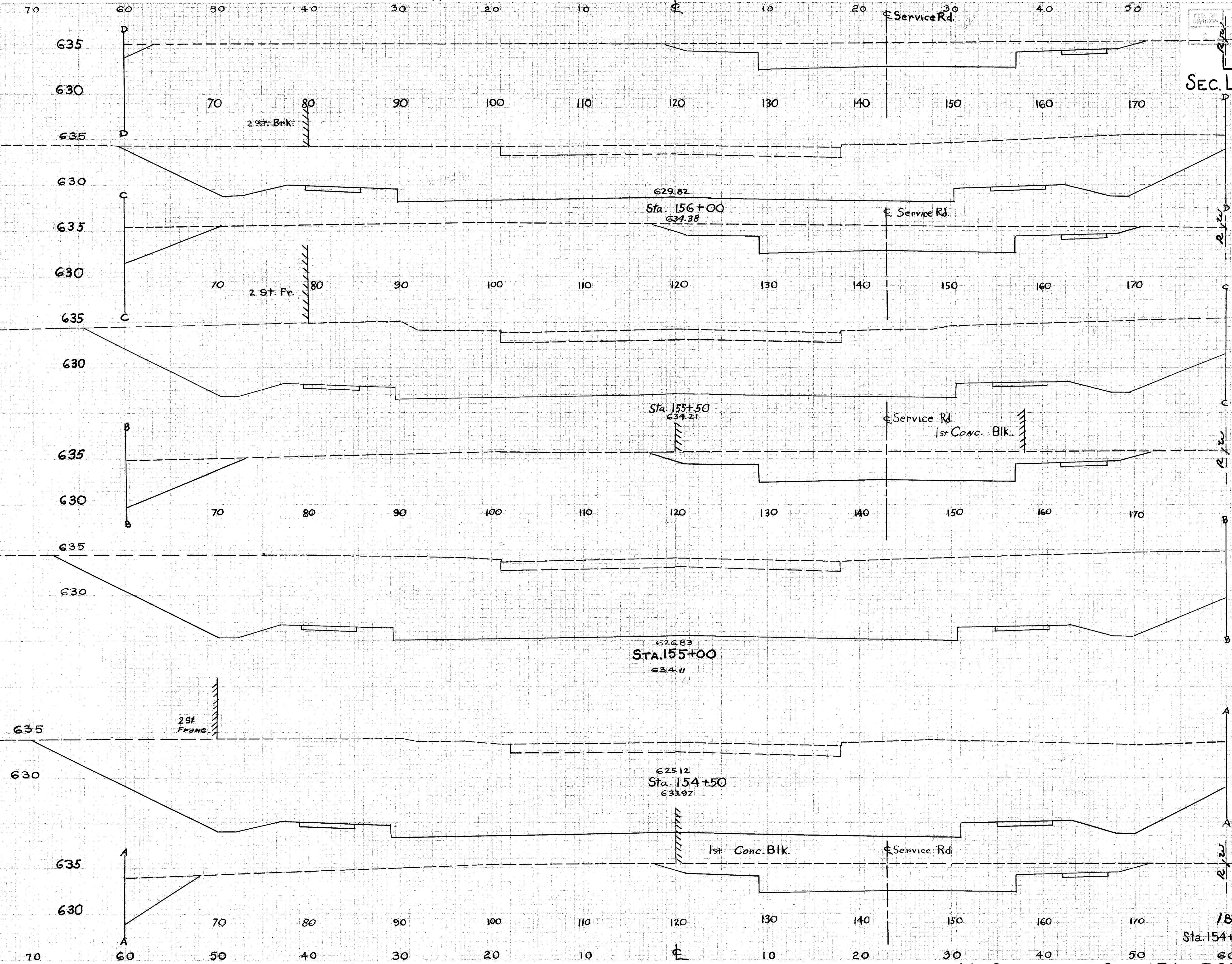
X-SECTIONS STA. 154+50 TO STA. 156+00
