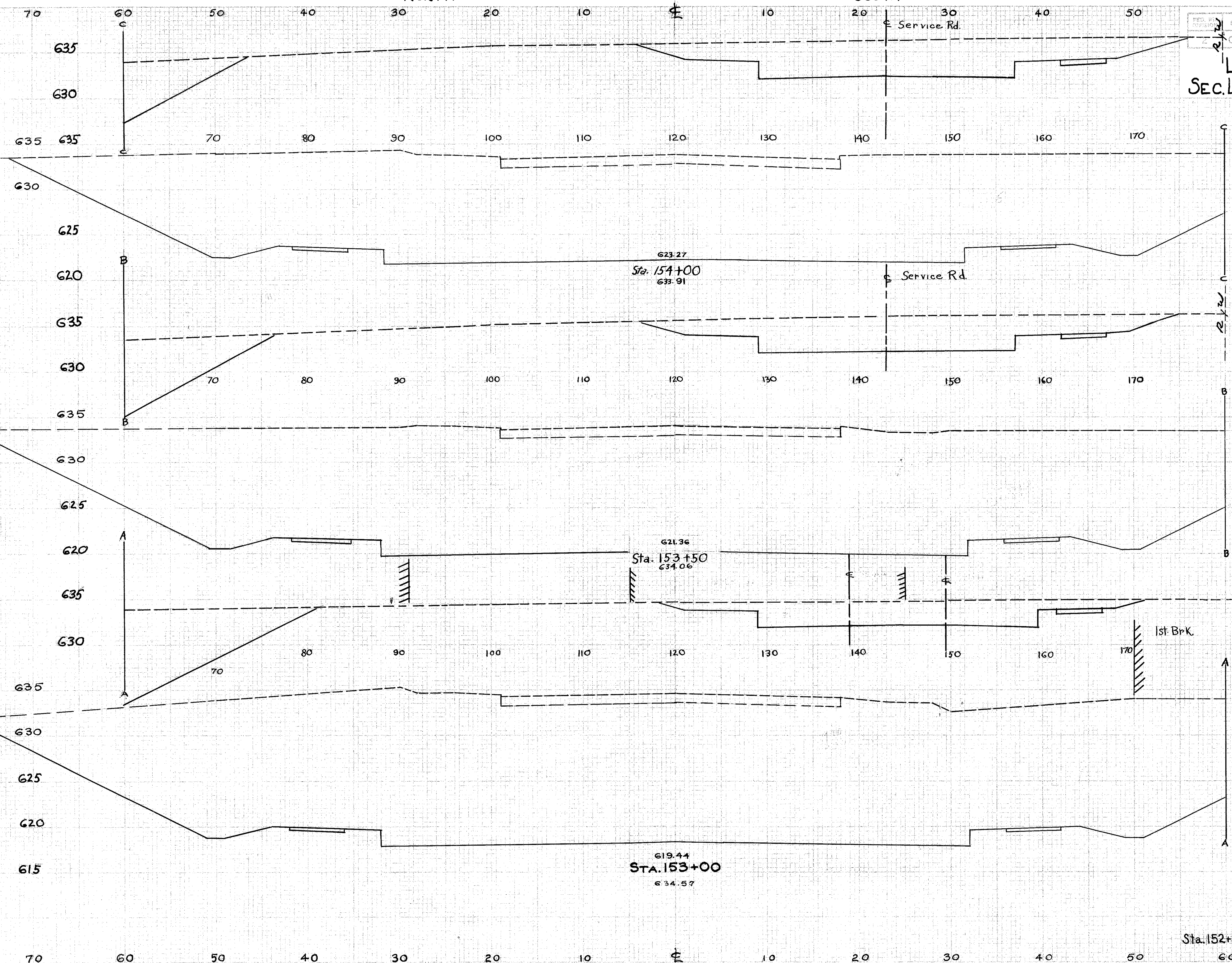
X-SECTIONS STA. 153+00 TO STA. 154+00
