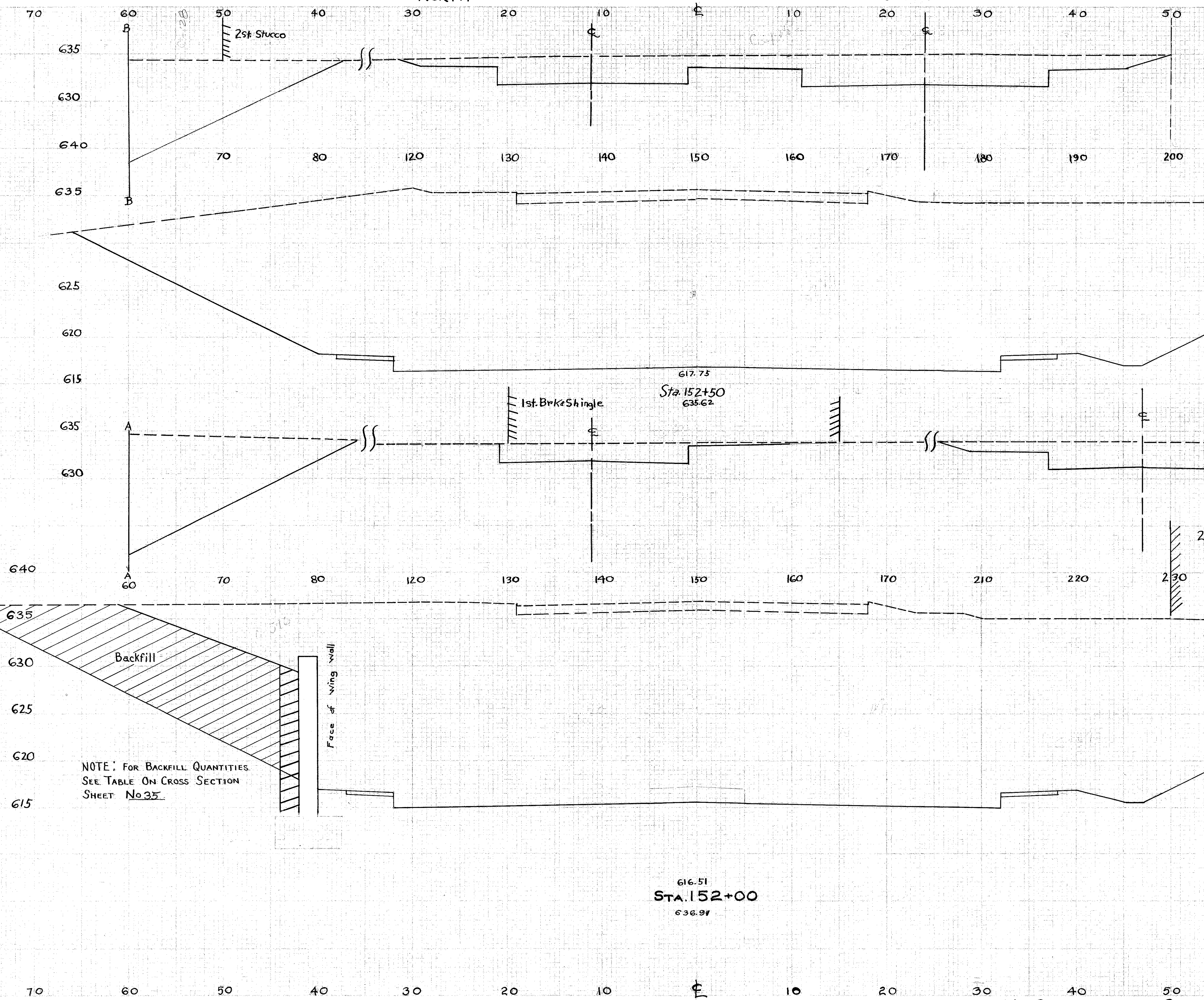
X-SECTIONS STA. 152+00 TO STA. 152+50
