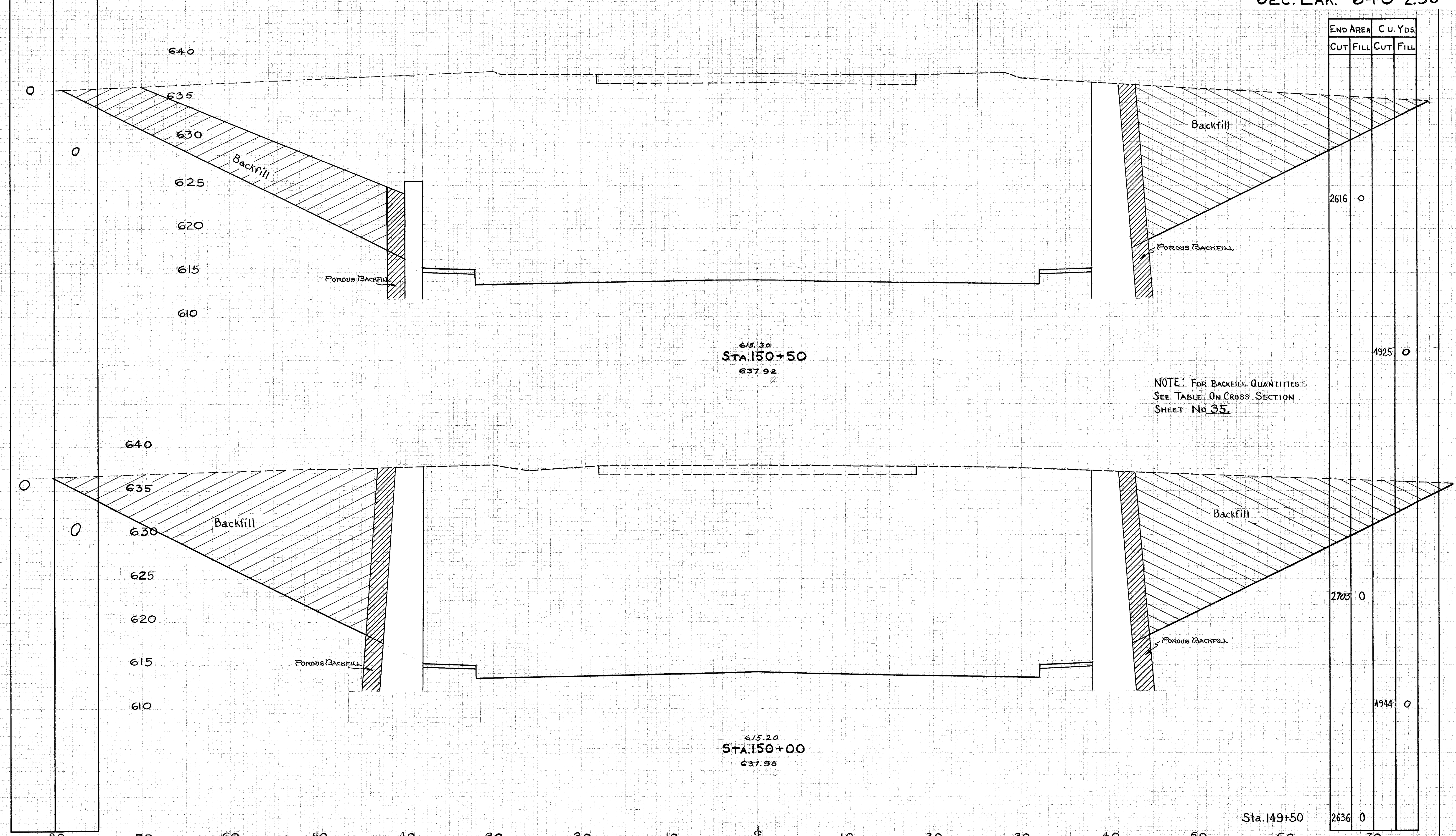
X-SECTIONS STA. 150+00 TO STA. 150+50
