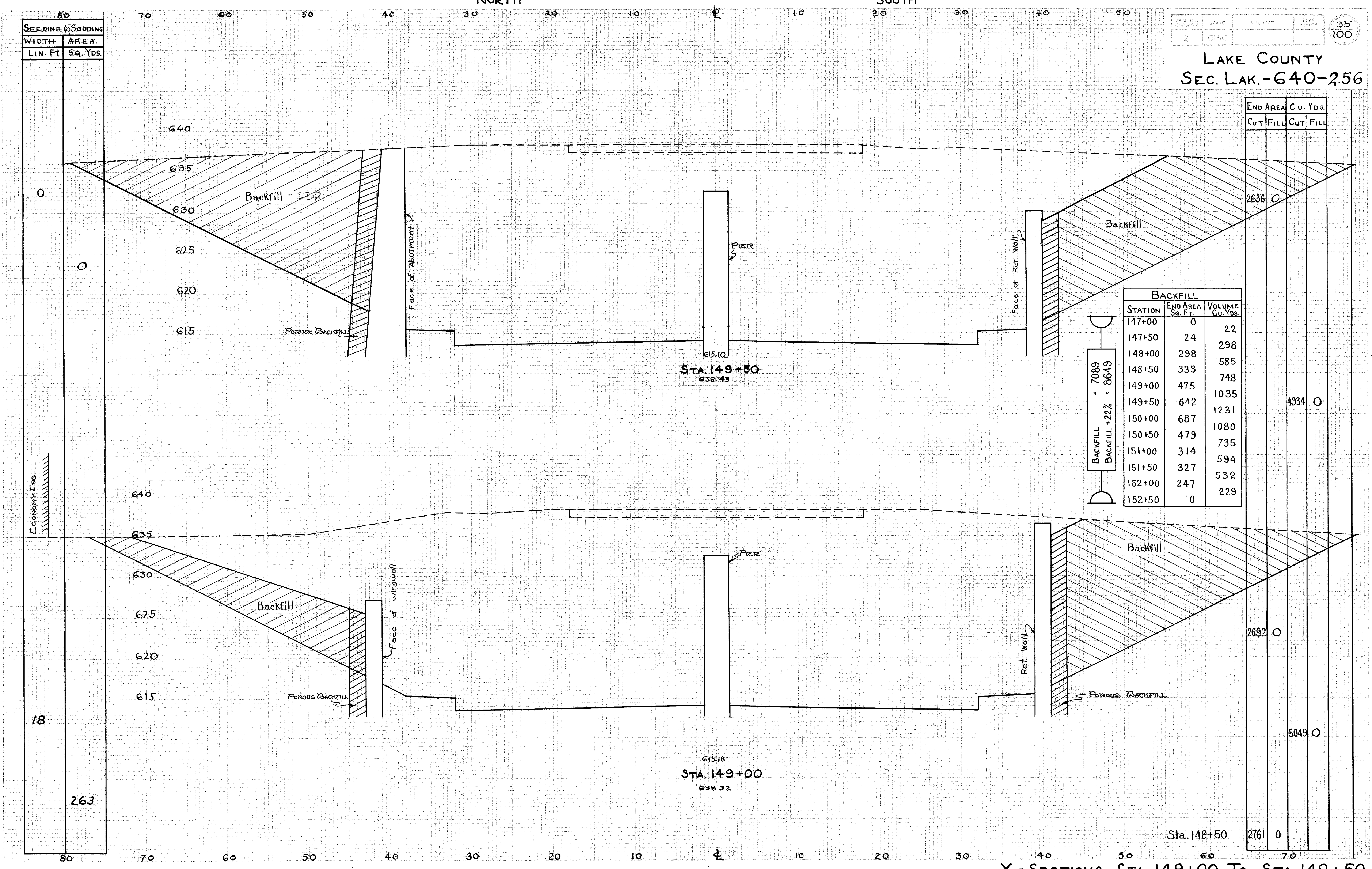
X-SECTIONS STA. 149+00 To STA. 149+50
