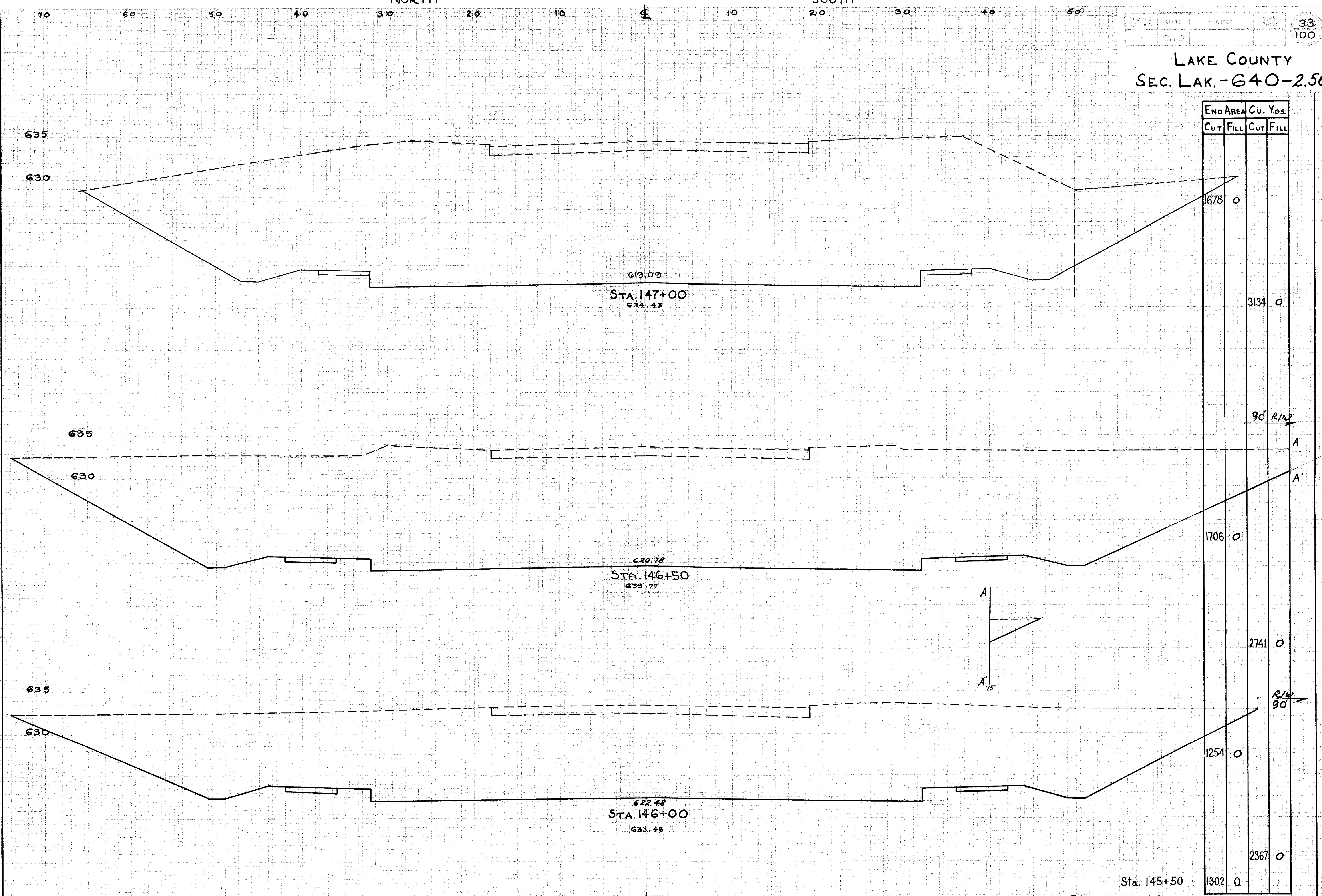
X-SECTIONS STA. 146+00 TO STA. 147+00
