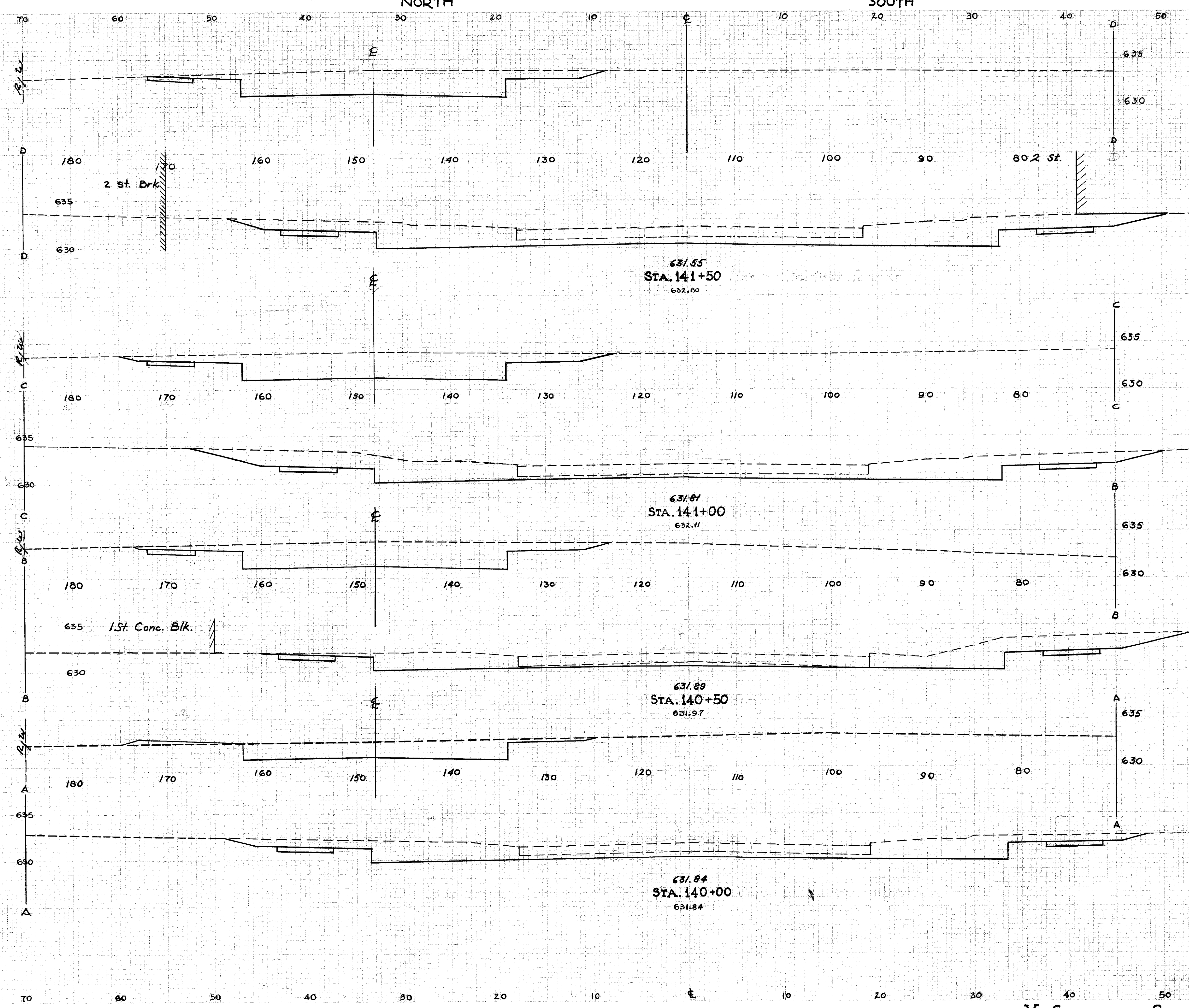
X-SECTIONS STA. 140+00 TO STA. 141+50
