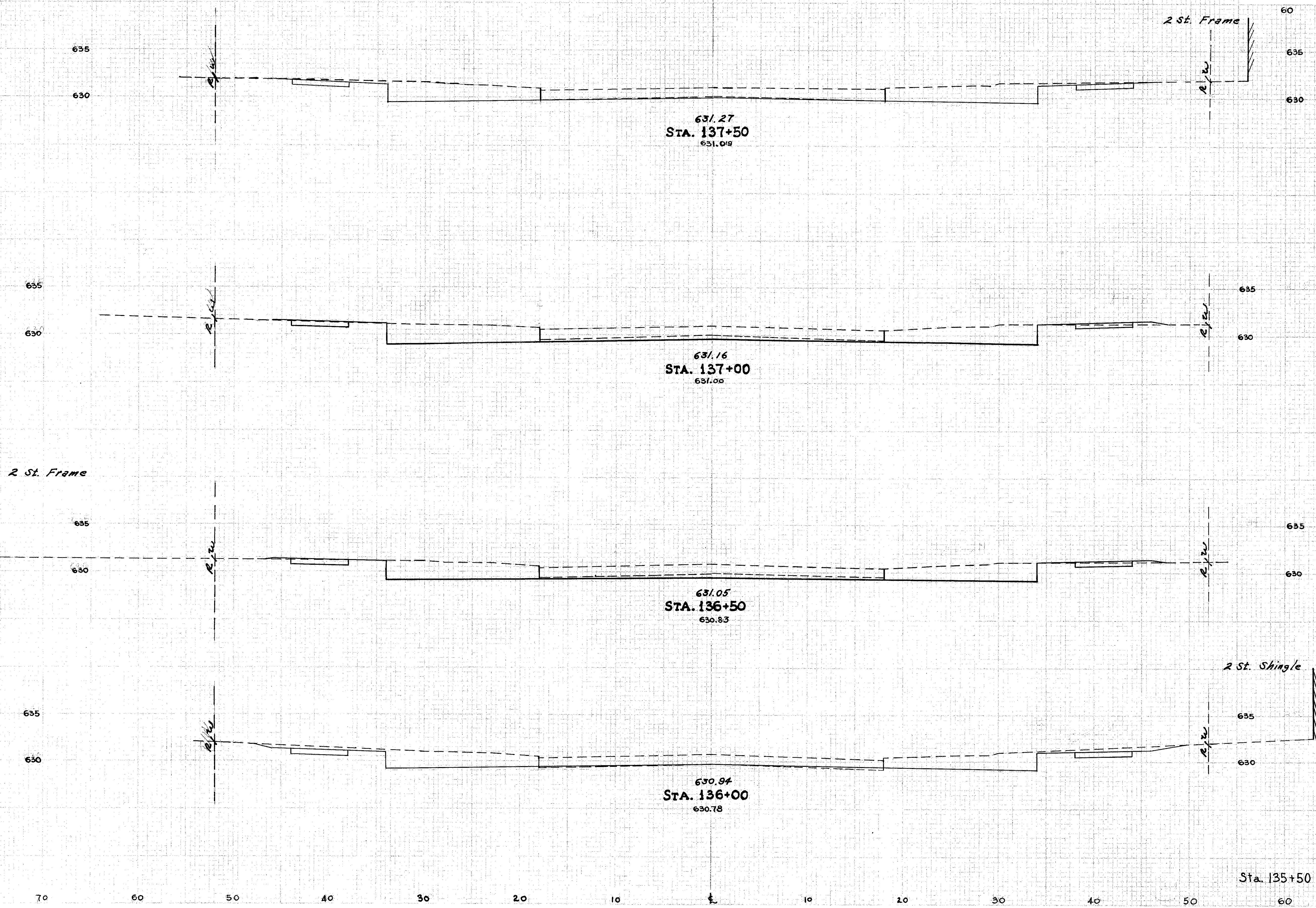
X-SECTIONS STA. 136+00 TO STA. 137+50
